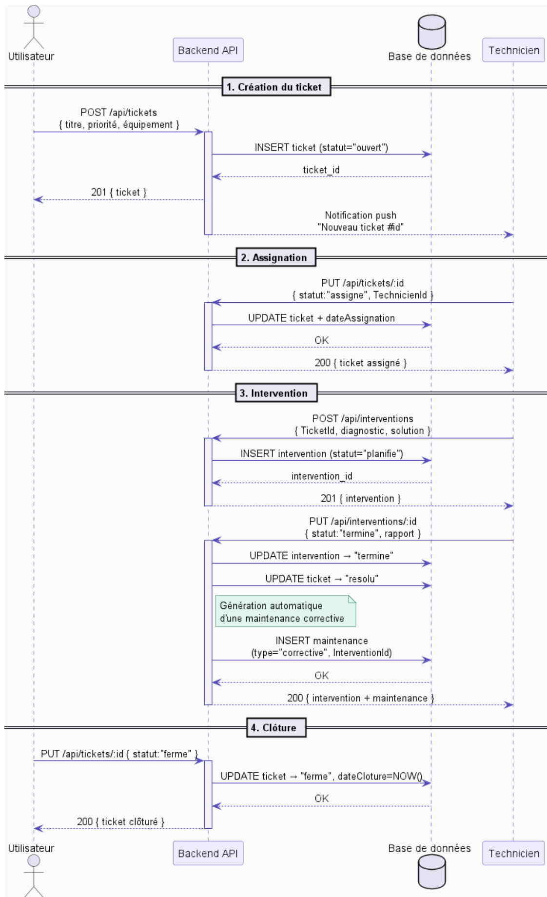
FIGURE 3.5 – Diagramme de séquence global
