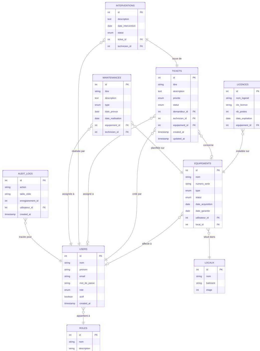
FIGURE 5.2 – Diagramme entité-relation de la base MySQL
