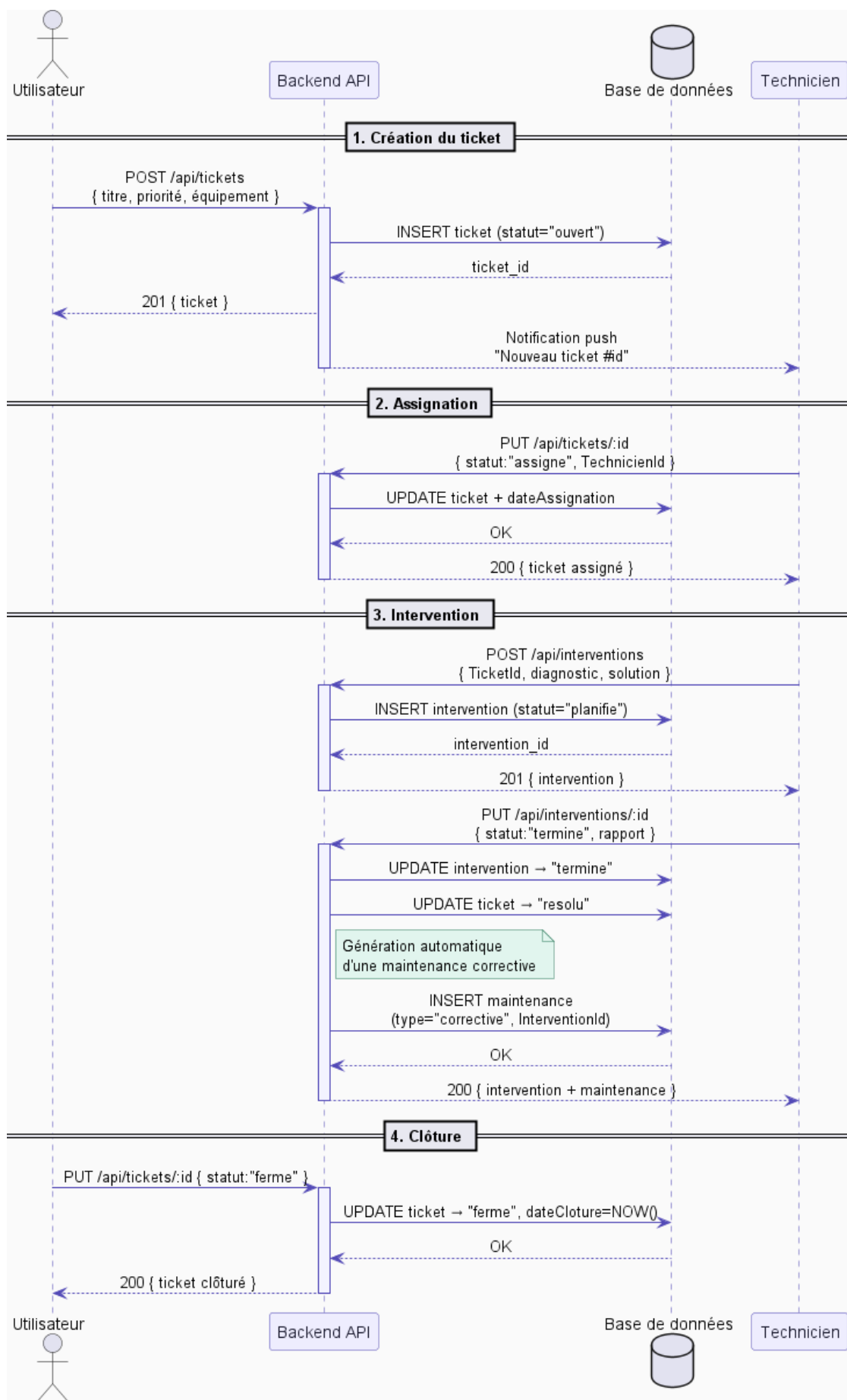
FIGURE 3.5 – Diagramme de séquence global
