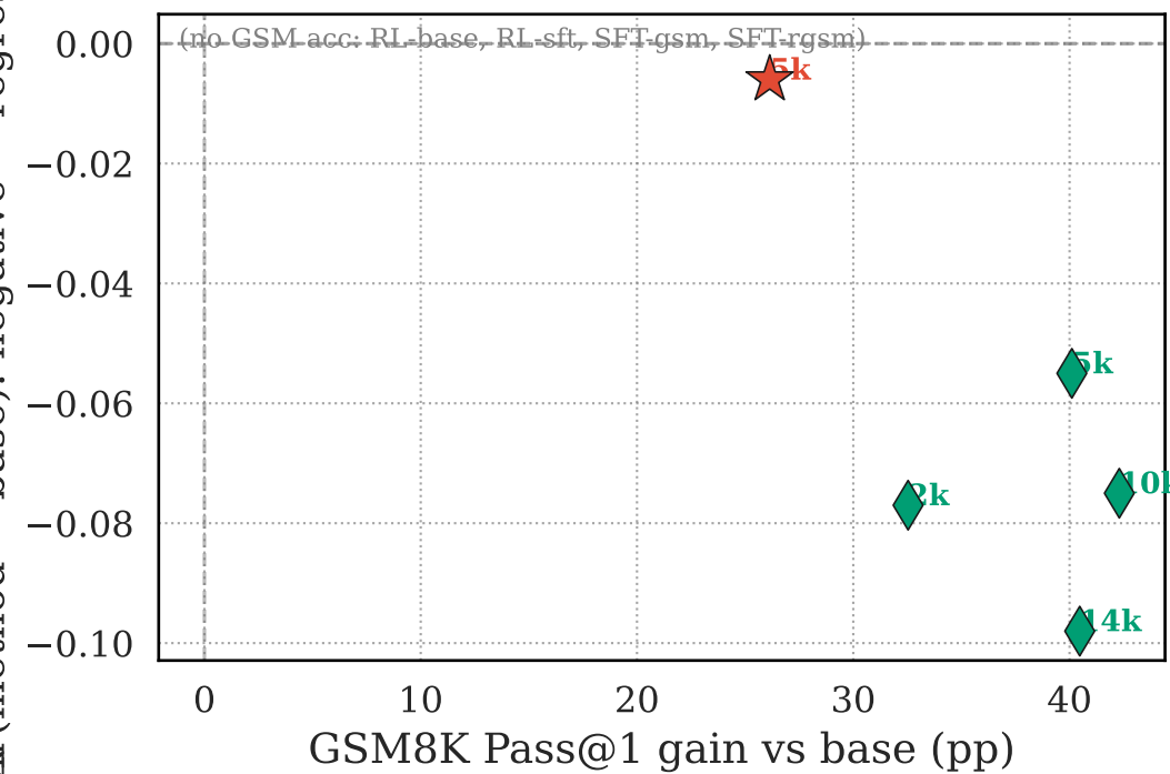
PIQA
