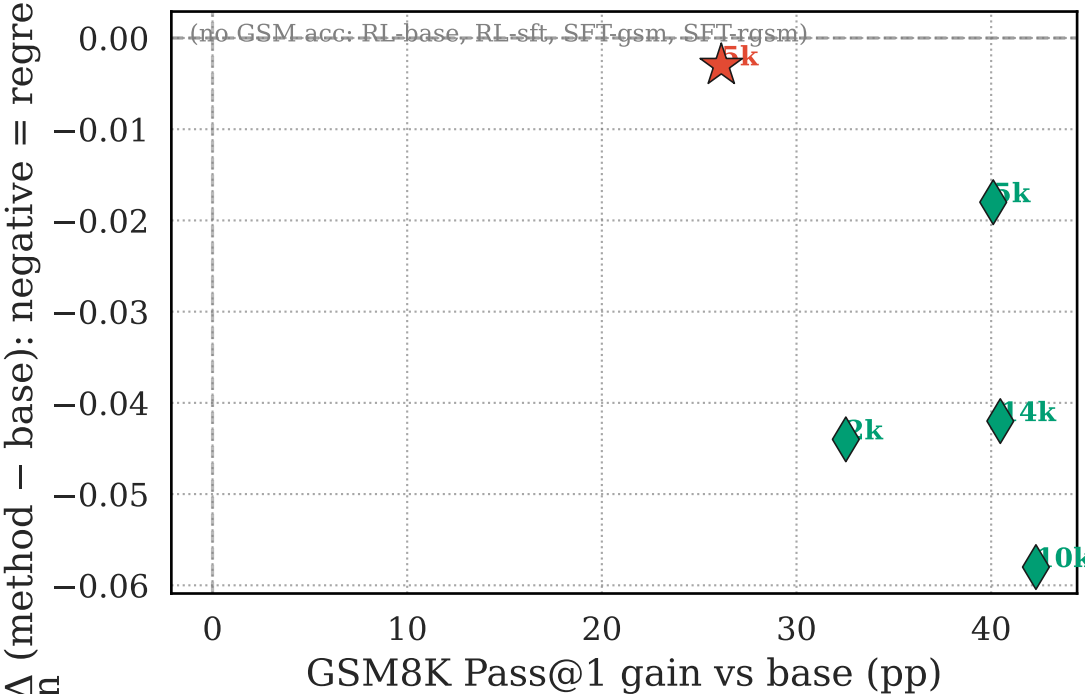
IFEval BPB
