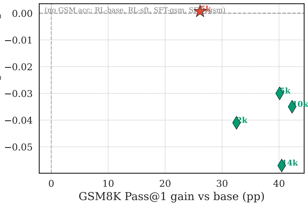
WinoGrande Acc
