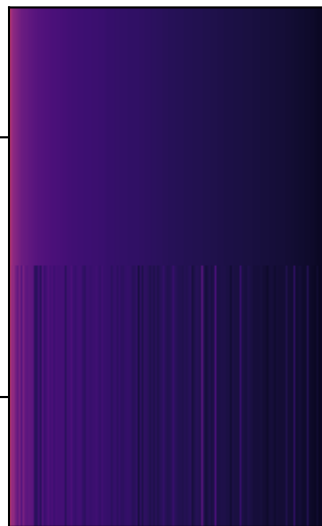
PeMS7_1026
