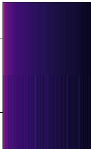
PeMS7_228
