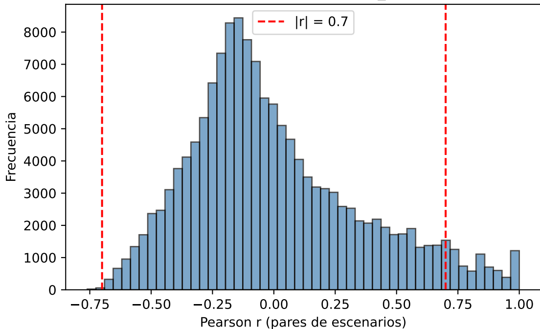
Distribución Pearson (reduced_17, d=17)
