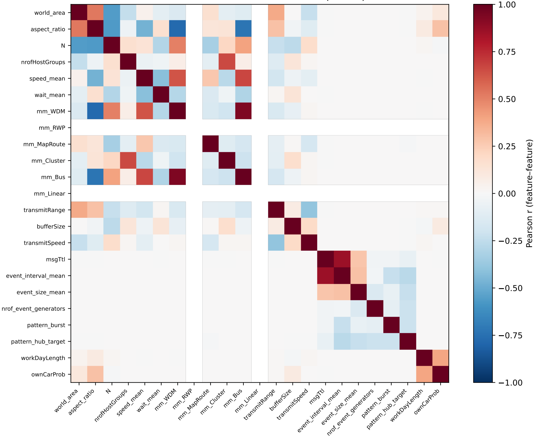
Correlación entre features del core (23x23)
