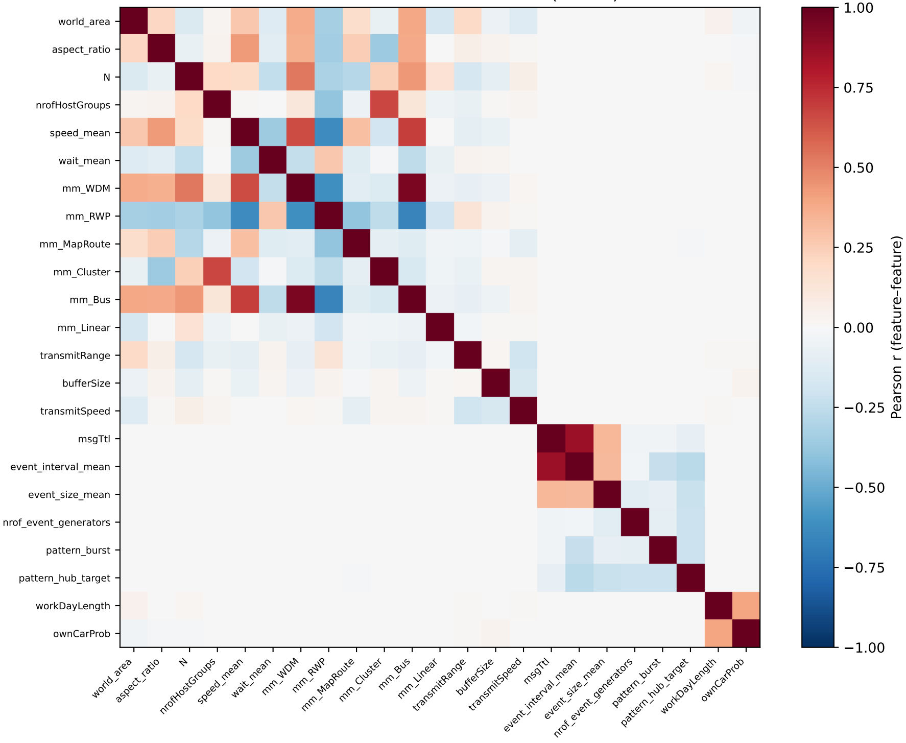
Correlación entre features del core (23×23)
