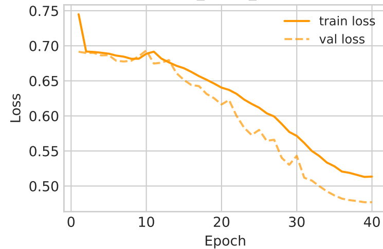
StandardCNN_allseq_undersample
