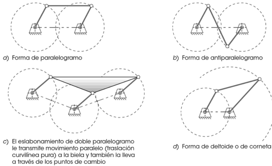
Figura 2.1: Inversiones del caso especial de Grashof [14].
