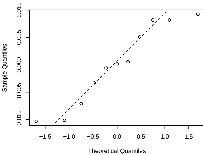
QQ-plot dos resíduos
