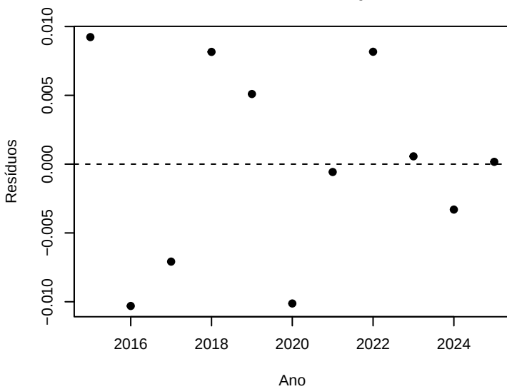
Resíduos vs Tempo
