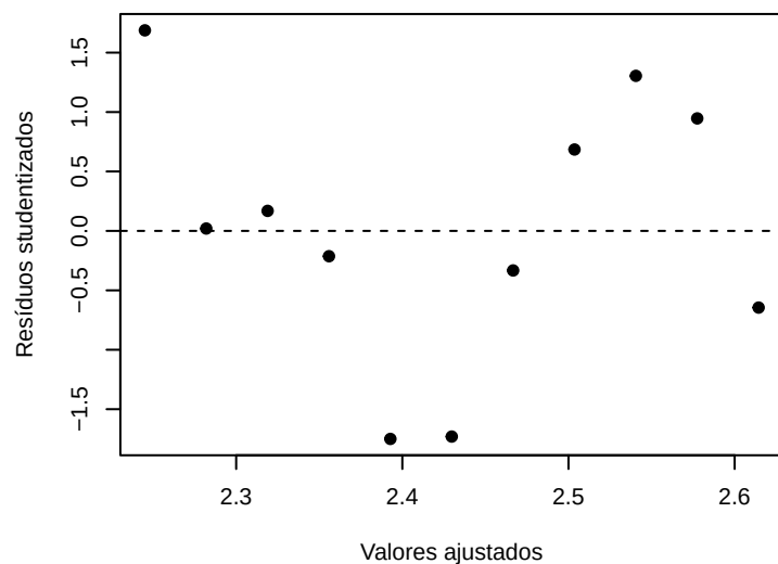
Resíduos studentizados vs Ajustados
