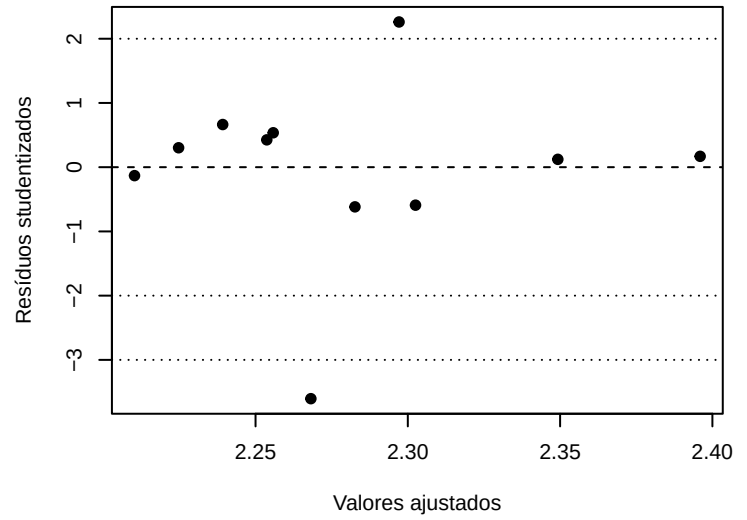
Resíduos studentizados vs Ajustados
