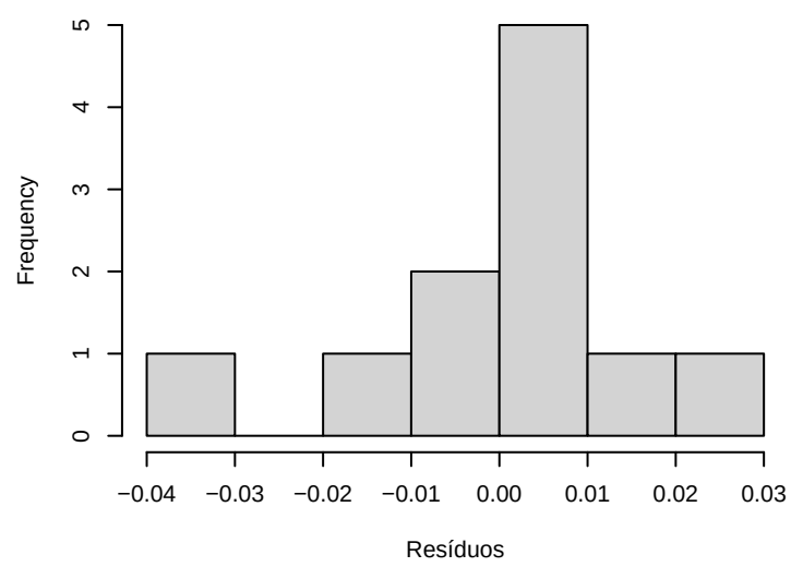
Histograma dos resíduos
