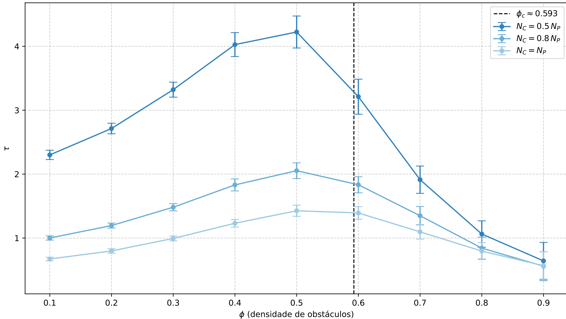
\tau vs \phi — modelo EXP \beta (3 cenários)
