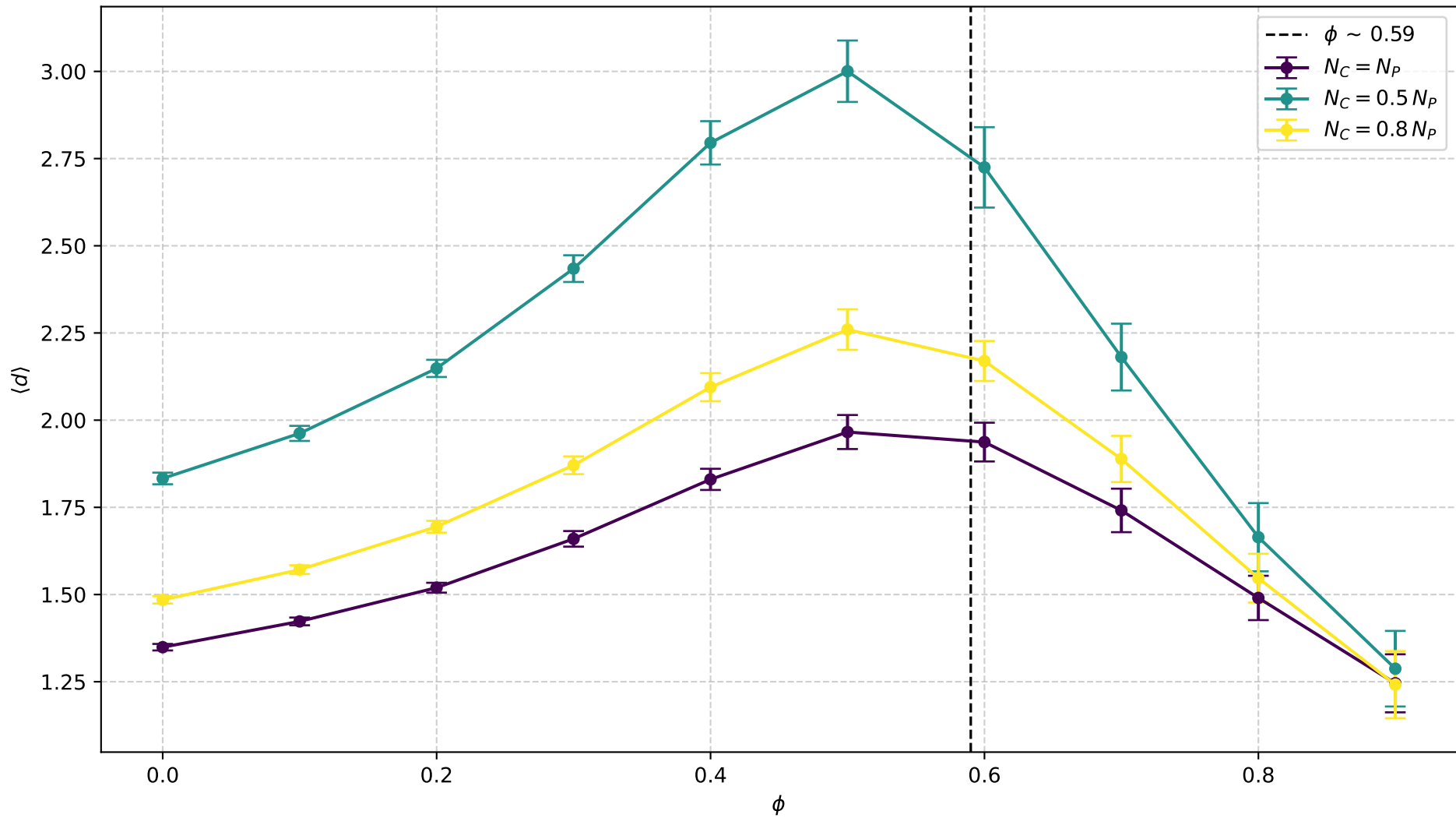
\langle d \rangle (presa \rightarrow caçador) vs \phi — N_C = N_P vs N_C = 0.5 N_P
