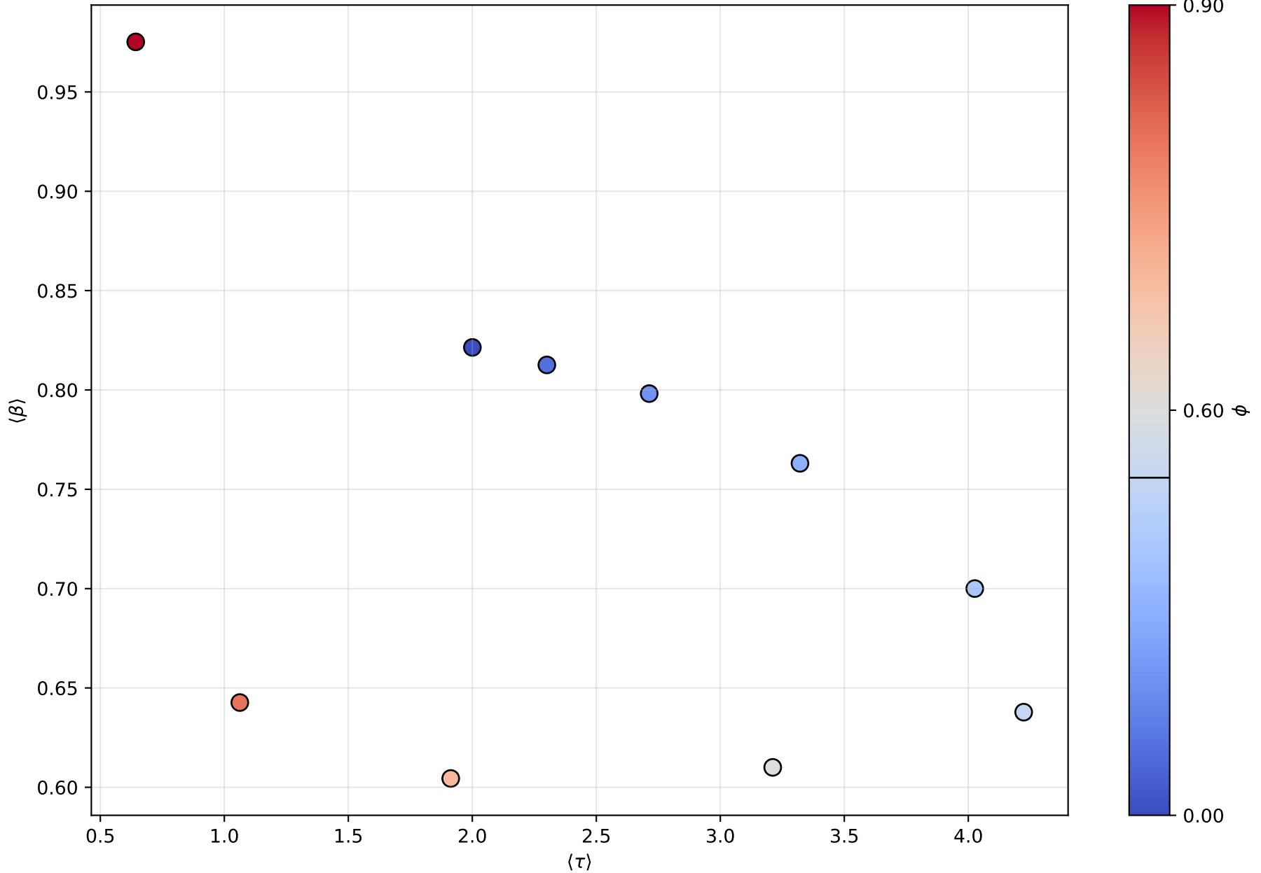
Média de \beta em função de \tau , Nc = Np * 0.5
