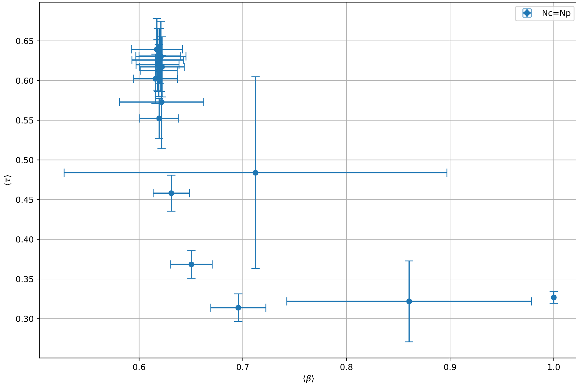
Média de \tau em função de \beta
