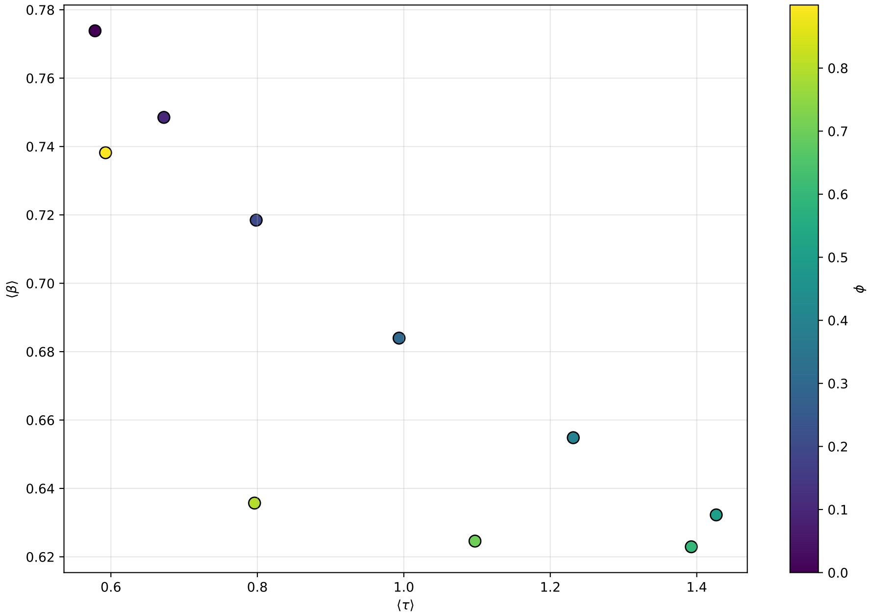
Média de \beta em função de \tau
