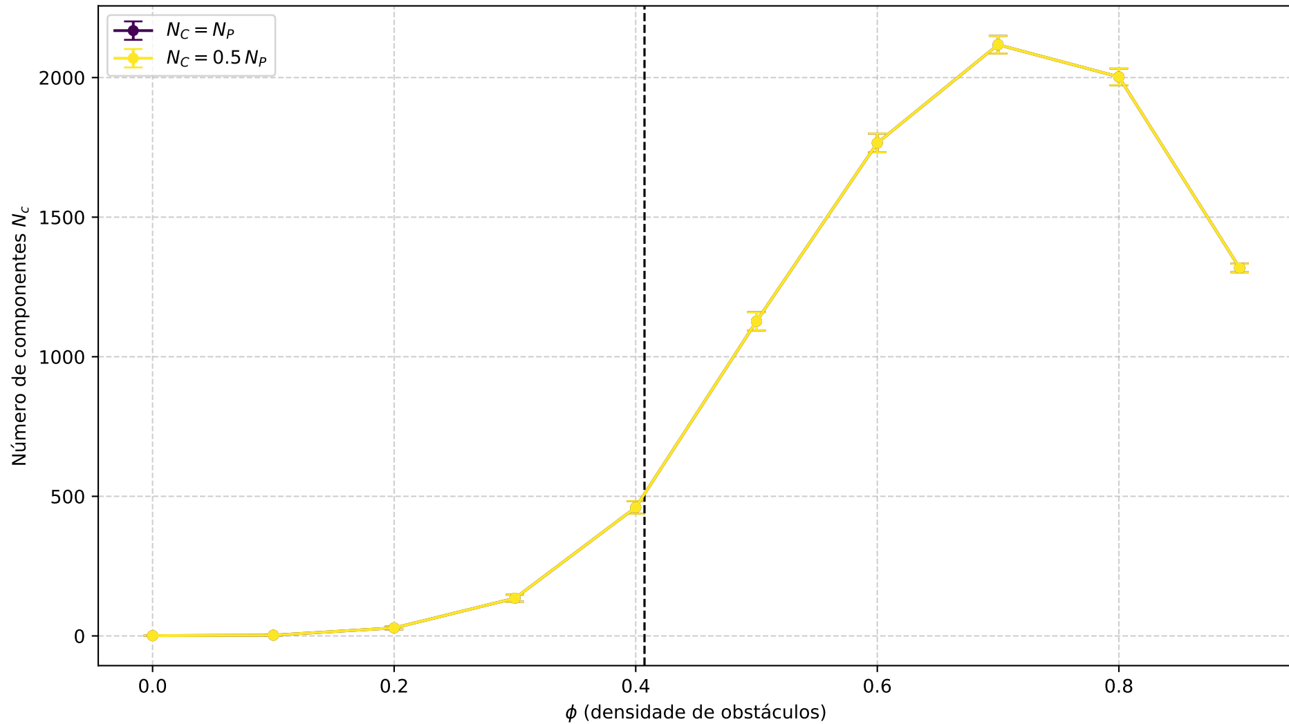
Fragmentação do espaço livre: N_c vs \phi
