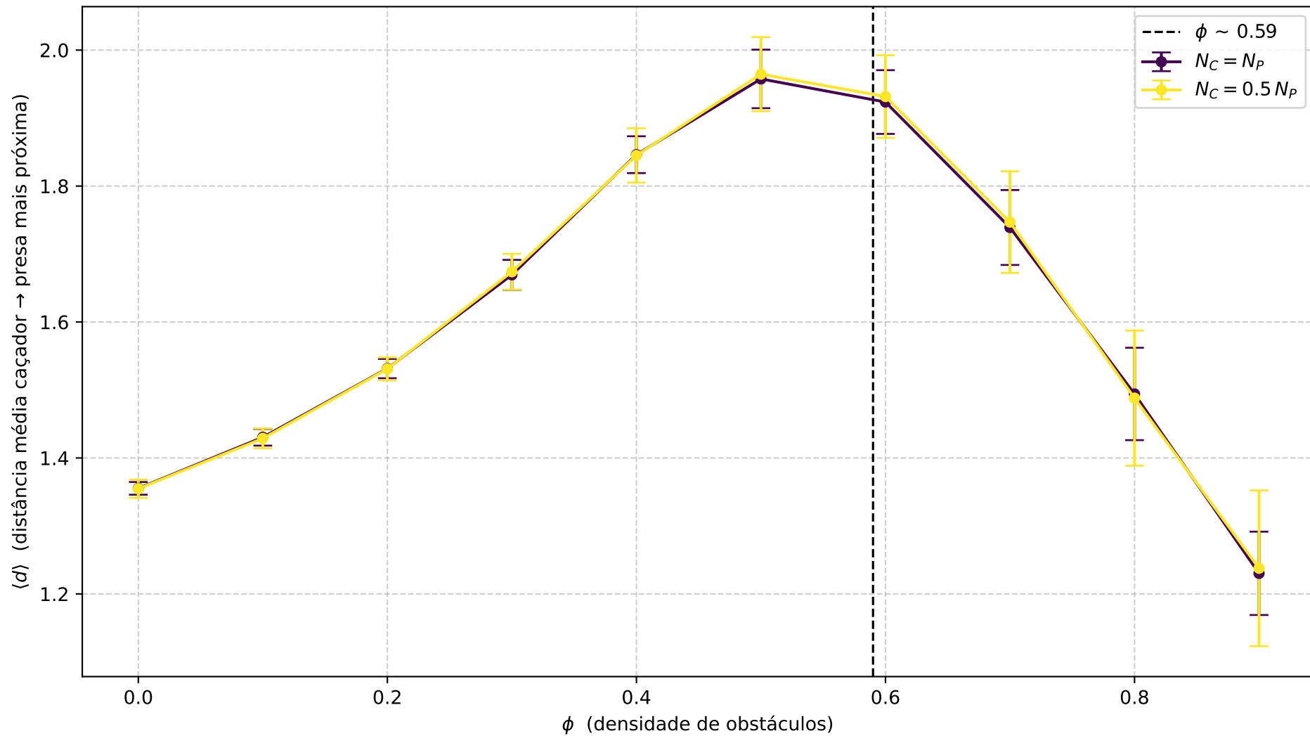
Distância média \langle d \rangle vs \phi — N_C = N_P vs N_C = 0.5 N_P
