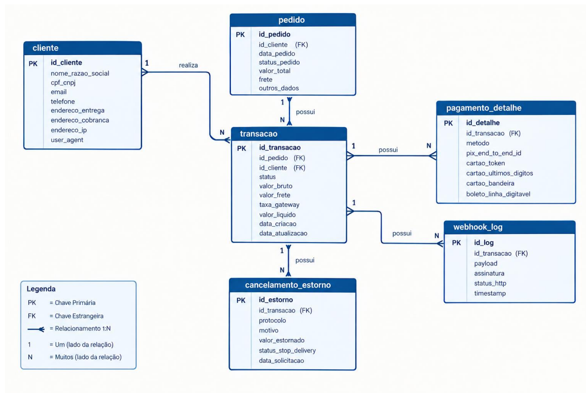
Figura 2: Modelo DER das Transações de compra.
