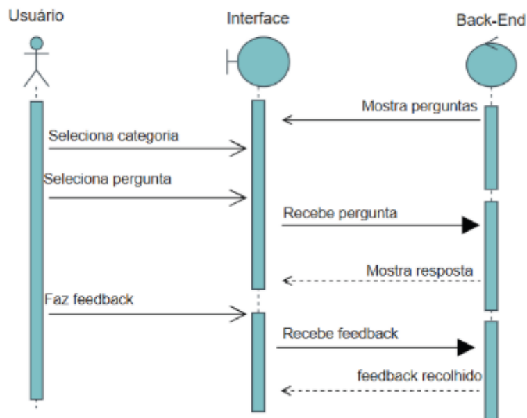
Figura 06, Diagrama de Sequência sobre perguntas e respostas automáticas do sistema
