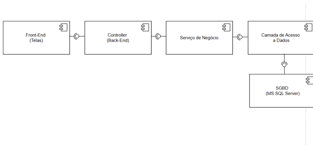
Figura 10, Diagrama de Componentes para interações da plataforma
