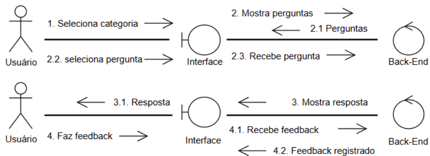
Figura 08, Diagrama de Colaboração sobre interações do Perguntas e Respostas Automáticas
