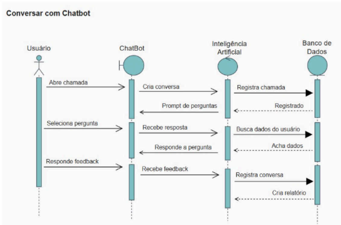
Figura 05, Diagrama de Sequência sobre a conversa do usuário no ChatBot
