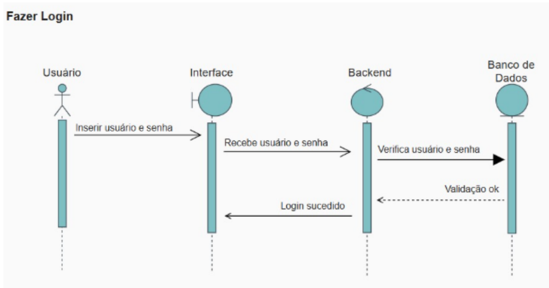
Figura 04, Diagrama de Sequência sobre o login de usuários
