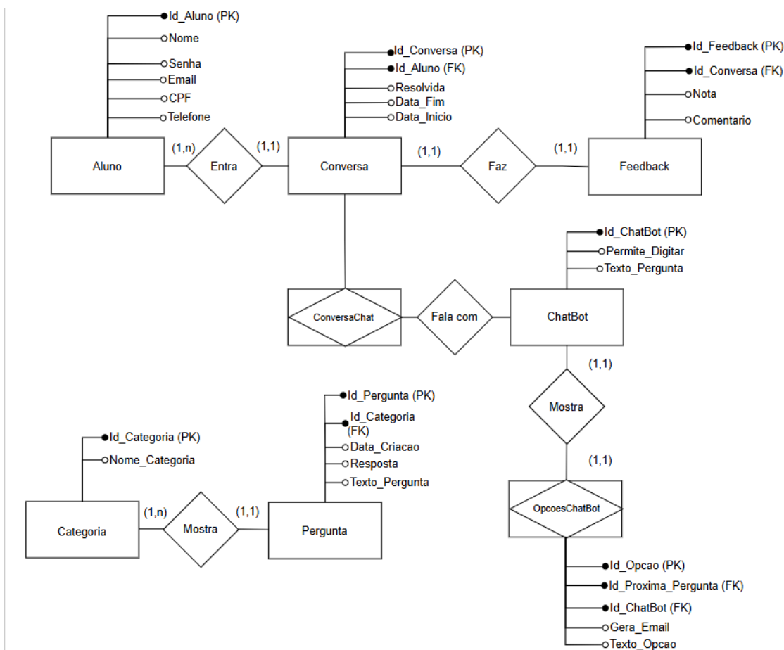
Figura 28, Diagrama de Entidade-Relacionamento
