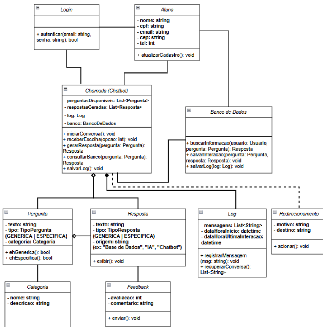
Figura 02, Diagrama de Classe sobre as funcionalidades do sistema
