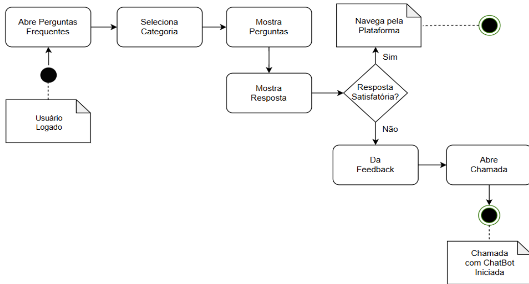
Figura 12, Diagrama de Atividades para interações do chatbot com o usuário
