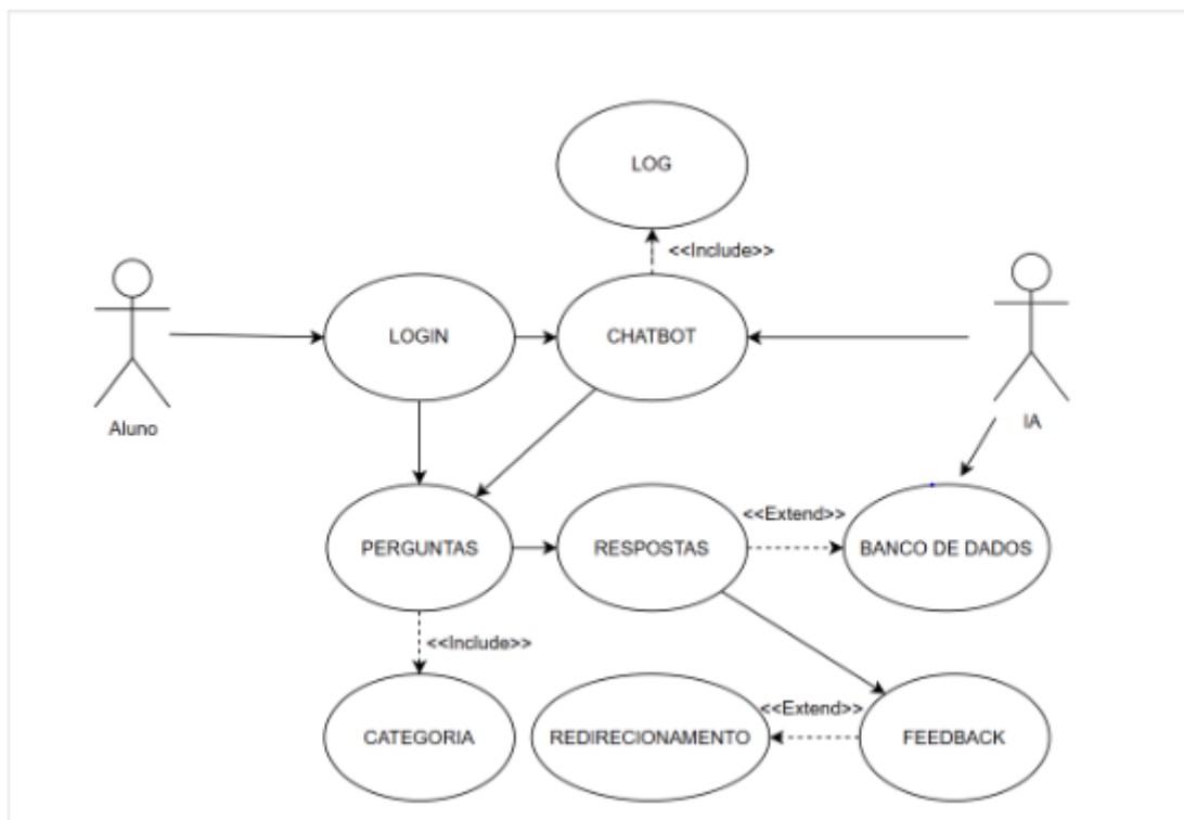
Figura 01, Diagrama de Casos de Uso sobre as funções dos atores do software
