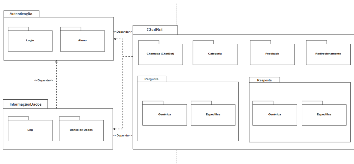
Figura 03, Diagrama de Pacote sobre funcionalidades do sistema
