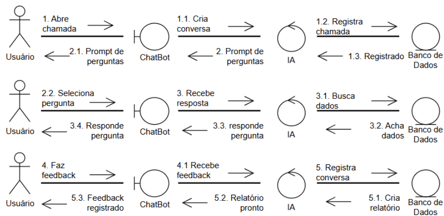
Figura 09, Diagrama de Colaboração sobre interações do Conversar com ChatBot
