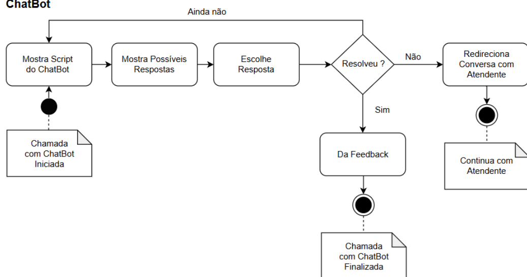
Figura 13, Diagrama de Atividades para interações com as perguntas automáticas.
