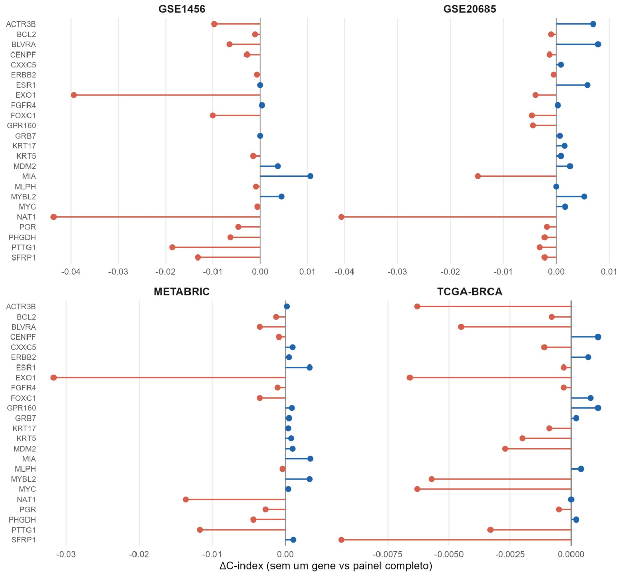
Figura 9 — Análise de sensibilidade leave-one-gene-out. Cada barra mostra a mudança no C-index OOF após remoção individual de cada gene CorePAM. Nenhuma remoção causa perda catastrófica (máximo |\Delta C| = 0,044 ), demonstrando distribuição equilibrada da informação prognóstica.
