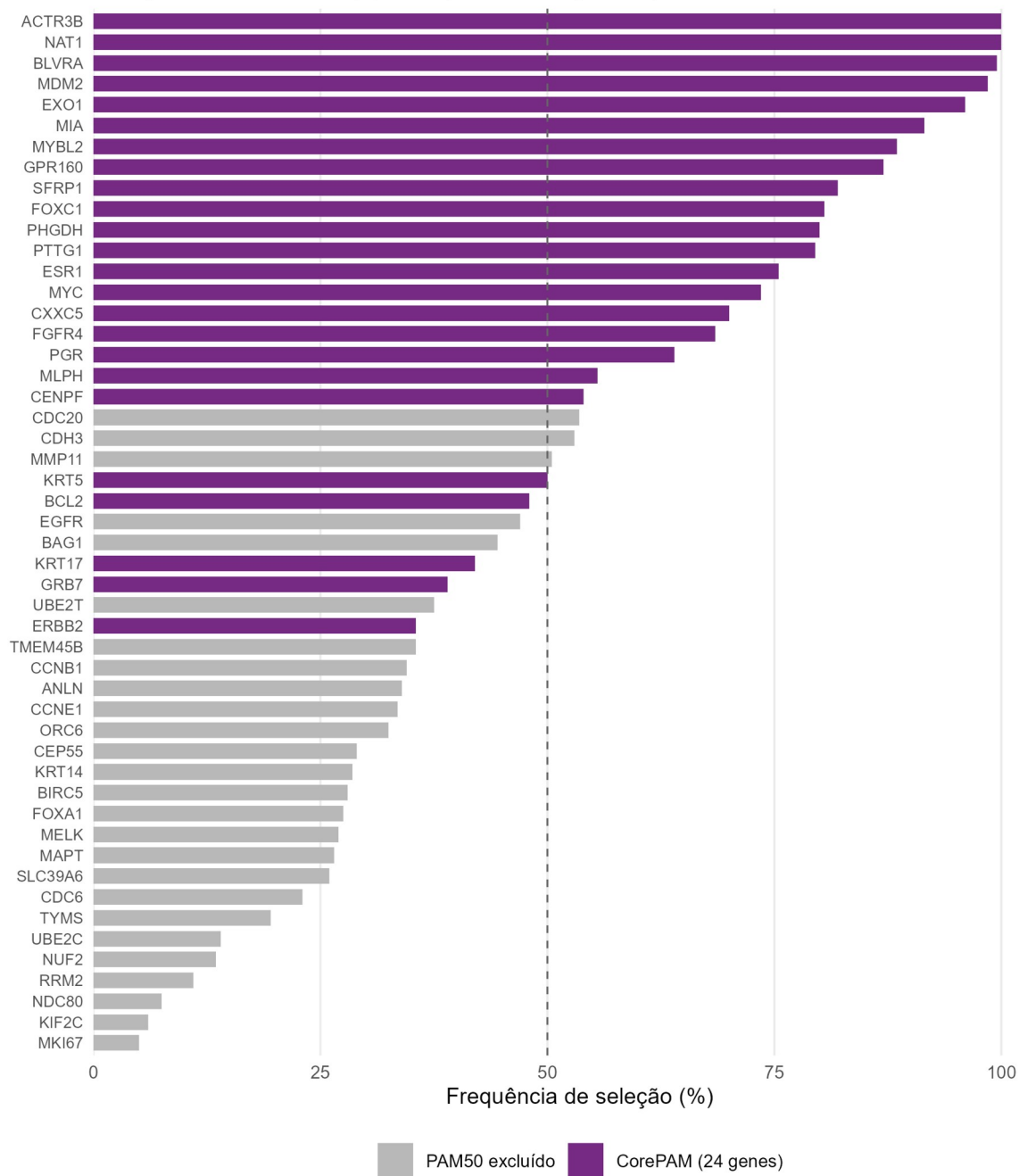
Figura 8 — Estabilidade bootstrap da seleção de genes (B = 200 reajustes no SCAN-B). Cada barra representa a frequência com que um gene foi selecionado nas reamostras. 15 dos 24 genes CorePAM foram selecionados em pelo menos 70% das iterações, com ACTR3B e NAT1 a 100% e frequência mínima de 35,5%.
