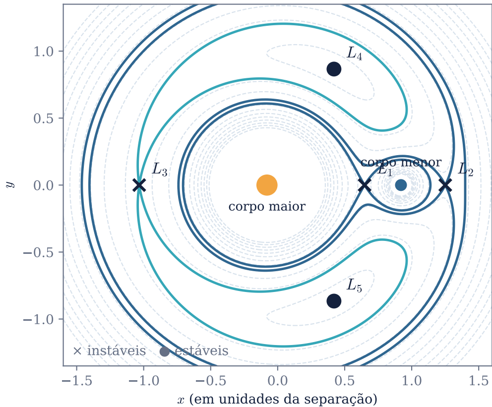
(a) o potencial efetivo, no referencial girante
