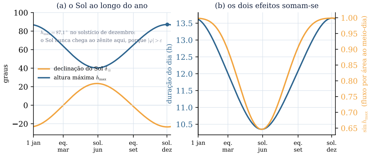
Figura 2: Por que existem estações, em números, para Joinville. (a) A declinação do Sol varia entre \pm\varepsilon ao longo do ano, e com ela a altura máxima h_{\max} = 90^\circ - |\varphi - \delta_\odot| . Como |\varphi| = 26,3^\circ excede a obliquidade, o Sol nunca alcança o zênite aqui: no solstício de dezembro ele para a 87,1^\circ . (b) Os dois efeitos caminham juntos e no mesmo sentido: no verão o dia dura mais (13,6 h contra 10,4 h no inverno) e cada metro quadrado recebe mais fluxo ao meio-dia, porque \sin h_{\max} é maior. É a soma dos dois, e não a distância ao Sol, que produz as estações.
