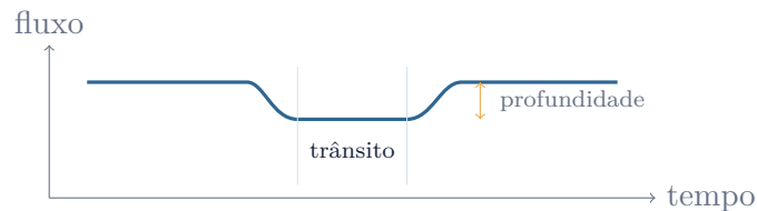
Figura 9: Curva de luz de trânsito. A queda de brilho mede principalmente a razão entre o raio do planeta e o raio da estrela.
