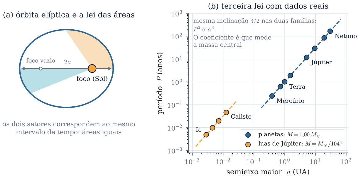
Figura 8: As leis de Kepler. (a) Órbita de excentricidade 0,55 obtida resolvendo a equação de Kepler M = E - e \sin E . O corpo central ocupa um foco, o outro fica vazio, e os dois setores sombreados — percorridos no mesmo intervalo de tempo — têm a mesma área: perto do periélio o planeta corre mais e cobre um ângulo grande com raio curto; perto do afélio faz o oposto. (b) A terceira lei com dados tabelados: os oito planetas em torno do Sol e os quatro satélites galileanos em torno de Júpiter. As duas famílias caem sobre retas de mesma inclinação 3/2 mas coeficientes diferentes, e é o coeficiente que carrega a física: aplicando M = 4\pi^2 a^3 / GP^2 aos planetas obtém-se 1,00 M_{\odot} ; aplicando às luas, 1,90 \times 10^{27} \text{ kg} , a massa de Júpiter, cerca de M_{\odot}/1047 . A mesma lei, medindo dois corpos centrais diferentes.
