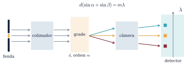
(a) o caminho da luz dentro de um espectrógrafo
