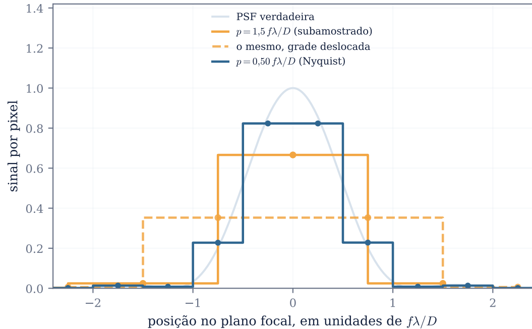
(a) subamostrado, a imagem depende de onde caem os pixels
