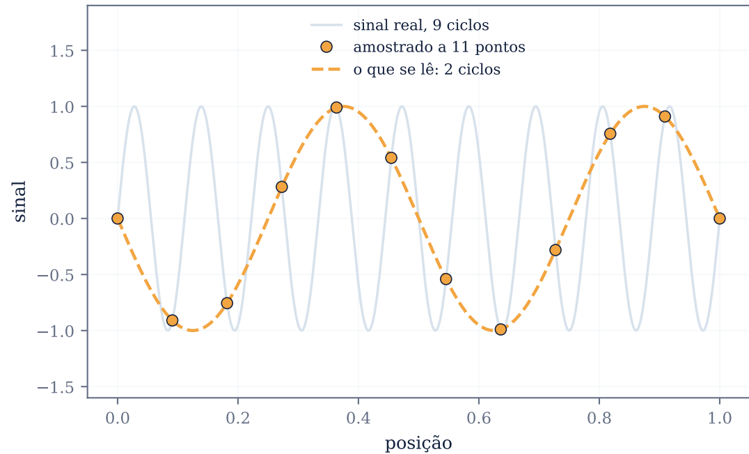
(b) abaixo de Nyquist, a frequência se disfarça
