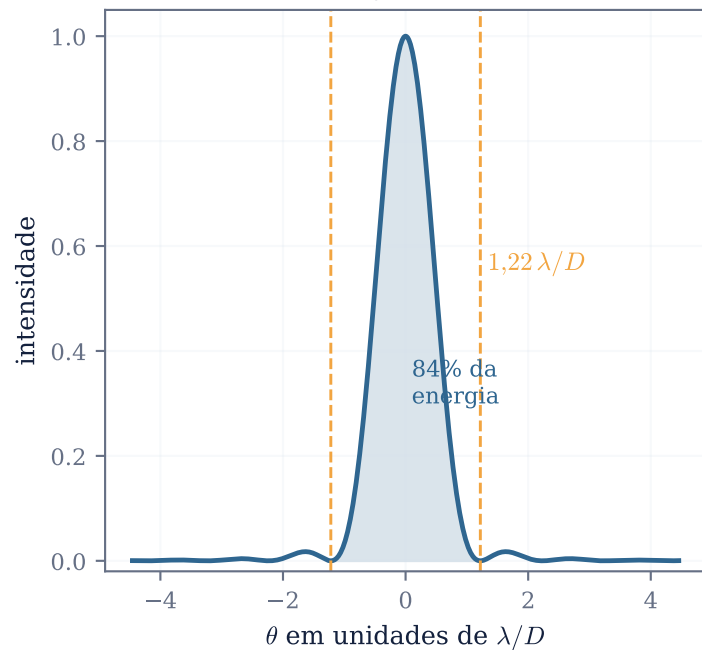
(a) o padrão de Airy
