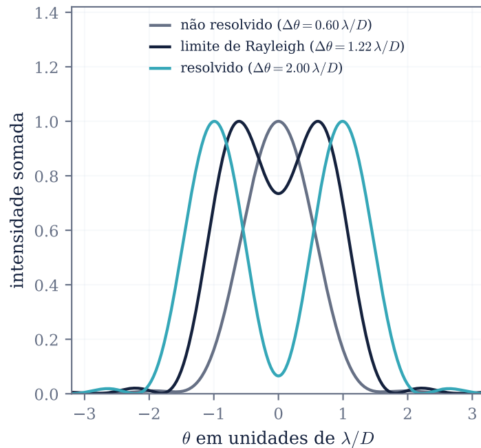
(b) duas fontes, três separações
