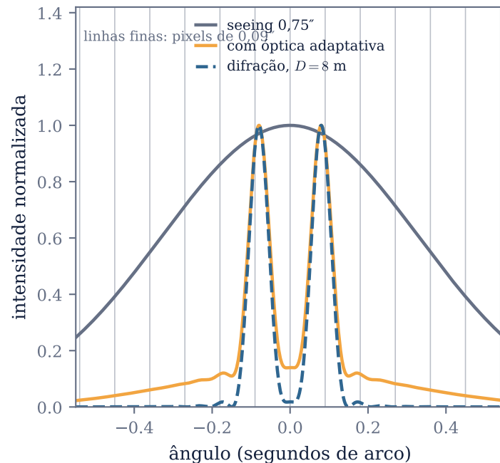
(c) duas fontes a 0,16" em 2,2 \mu\text{m}
