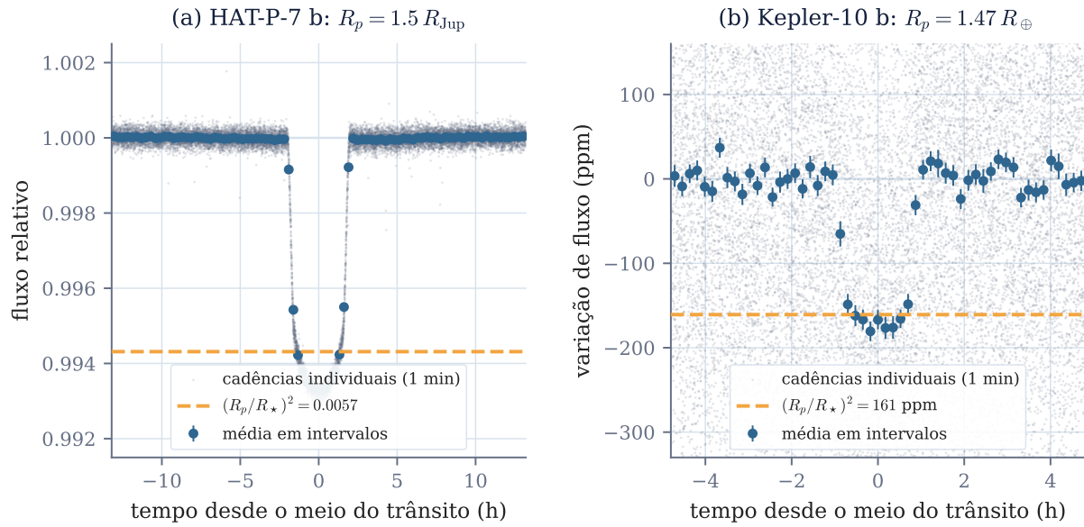
Figura 15: Curvas de luz de trânsito reais, medidas pelo Kepler. Fotometria de cadência curta (um ponto por minuto), dobrada no período orbital; os pontos cinza são cadências individuais e os círculos azuis são médias em intervalos de tempo. A linha tracejada não é ajuste algum: é a profundidade prevista por (R_p/R_\star)^2 com o raio do planeta e o raio da estrela medidos independentemente. (a) HAT-P-7 b, um Júpiter quente diante de uma estrela de 2 R_\odot : a queda é de 0,57% e o fundo achatado mostra o planeta inteiramente projetado sobre o disco estelar. (b) Kepler-10 b, um planeta rochoso de 1,5 R_\oplus : a queda é de apenas 161 partes por milhão, ou seja, 35 vezes menor, exatamente como a razão dos raios ao quadrado prevê. É a mesma física nas duas escalas, e é por isso que a estatística de exoplanetas nasceu dominada por planetas grandes. Dados: arquivo público do Kepler (MAST); efemérides do NASA Exoplanet Archive.
