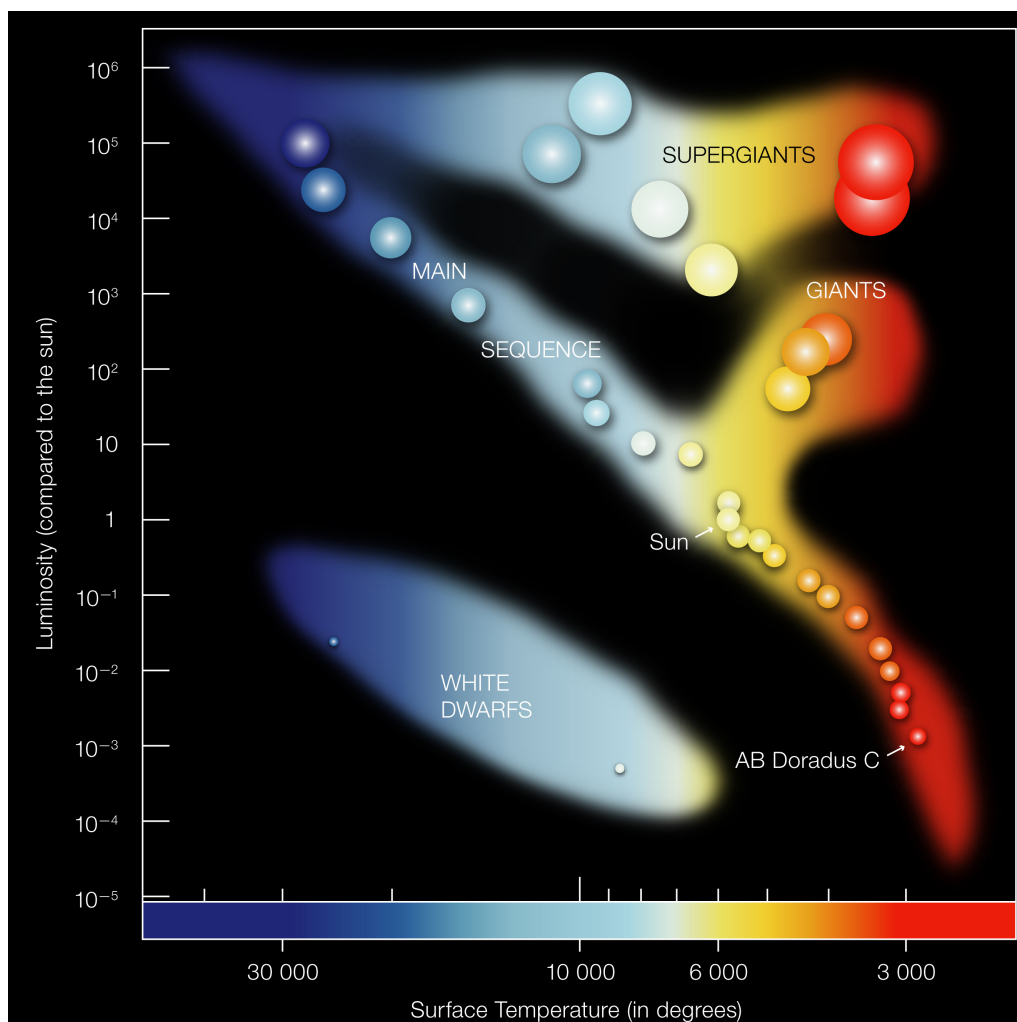
Figura 10: Diagrama Hertzsprung-Russell. Luminosidade (em unidades solares) contra temperatura efetiva, com o eixo de temperatura crescendo para a esquerda. A faixa diagonal é a sequência principal ( main sequence ); acima e à direita estão gigantes ( giants ) e supergigantes ( supergiants ), frias mas luminosas por terem raios enormes; abaixo e à esquerda estão as anãs brancas ( white dwarfs ), quentes mas pouco luminosas por terem raios pequenos. O tamanho dos círculos indica o raio relativo das estrelas. A posição de uma estrela combina temperatura, luminosidade, raio e estágio evolutivo. Crédito: ESO, licença CC BY 4.0 (eso0728c).
