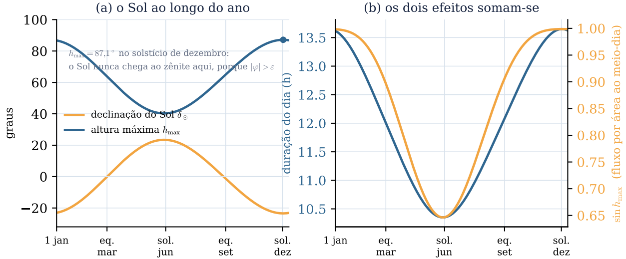
Figura 3: Por que existem estações, em números, para Joinville. (a) A declinação do Sol varia entre \pm\varepsilon ao longo do ano, e com ela a altura máxima h_{\max} = 90^\circ - |\varphi - \delta_{\odot}| . Como |\varphi| = 26,3^\circ excede a obliquidade, o Sol nunca alcança o zênite aqui: no solstício de dezembro ele para a 87,1^\circ . (b) Os dois efeitos caminham juntos e no mesmo sentido: no verão o dia dura mais (13,6 h contra 10,4 h no inverno) e cada metro quadrado recebe mais fluxo ao meio-dia, porque \sin h_{\max} é maior. É a soma dos dois, e não a distância ao Sol, que produz as estações.
