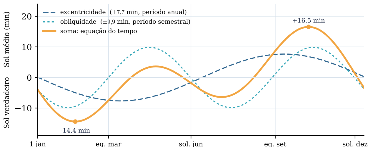
Figura 4: A equação do tempo e suas duas causas. A curva dourada é a diferença entre o Sol verdadeiro e o Sol médio, calculada a partir das duas expressões deduzidas acima. A componente da excentricidade (tracejada longa) tem período anual e amplitude 7,7 minutos; a da obliquidade (tracejada curta) tem período semestral e amplitude 9,9 minutos. A soma, com as fases reais, vai de -14,4 minutos em meados de fevereiro a +16,5 minutos no início de novembro. Duas propriedades geométricas independentes deixam sua assinatura em um único gráfico observável — e é por isso que um relógio de sol precisa de tabela de correção.
