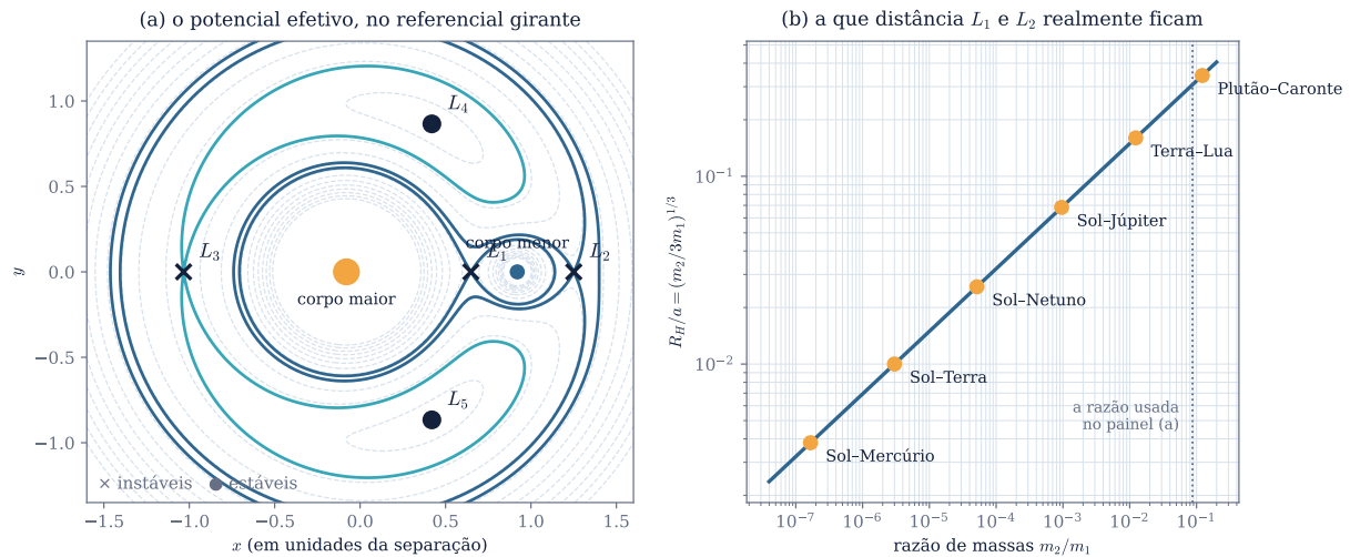
Figura 12: O potencial efetivo e os cinco pontos de Lagrange. (a) Curvas de nível de \Phi_{\text{ef}} no referencial girante. As destacadas passam por L_1, L_2, L_3 e L_4 : são as fronteiras das regiões proibidas, e é por isso que a de L_1 tem a forma de um oito — é ela que define os lóbulos de Roche. Os três pontos colineares são instáveis; L_4 e L_5 , nos vértices dos triângulos equiláteros, são estáveis. A razão de massas do desenho, m_2/m_1 = 0,087 , é muito maior que a real , senão L_1 e L_2 ficariam colados no corpo menor e invisíveis. (b) A escala verdadeira: a distância de L_1 e L_2 ao corpo menor é R_H/a = (m_2/3m_1)^{1/3} , e a raiz cúbica achata tudo — variar a razão de massas por seis ordens de grandeza move R_H/a por apenas duas. No sistema Sol-Terra, R_H/a = 0,010 : os telescópios em L_2 estão a 1,5 milhão de quilômetros, um centésimo da distância ao Sol.
