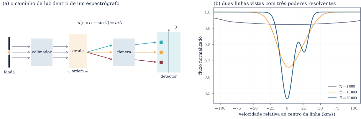
Figura 18: Espectrógrafo. (a) A fenda recorta uma faixa do campo; o colimador transforma o feixe divergente em paralelo; a grade dispersa cada comprimento de onda em um ângulo diferente; a câmera forma a imagem do espectro no detector. (b) Um par de linhas próximas, visto com três poderes resolventes. Em \mathcal{R} = 1000 há apenas uma depressão rasa; em 10 000, uma linha larga e assimétrica; em 60 000, as duas componentes aparecem separadas. A assimetria em resolução intermediária é o sinal de que há estrutura não resolvida — e é por isso que medir a posição do centro de uma linha exige saber do que ela é feita.
