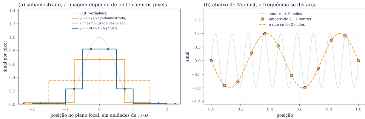
Figura 17: Por que o tamanho do pixel importa. (a) A mesma PSF registrada por dois detectores. Com p = 1,5 f\lambda/D o perfil medido depende de onde a grade de pixels calha de cair: deslocando-a por meio pixel, o valor de pico cai de 0,66 para 0,35 sem que nada tenha mudado no céu. Com p = 0,50 f\lambda/D — a condição de Nyquist — o perfil registrado é estável. (b) A versão unidimensional do mesmo fenômeno: um sinal de 9 ciclos amostrado em 11 pontos é lido como um sinal de 2 ciclos. A frequência alta não some; ela se disfarça de frequência baixa, e isso é aliasing .
