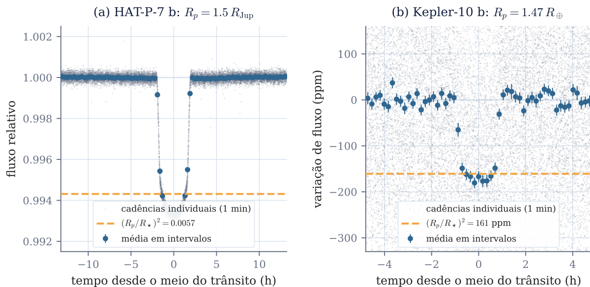
Figura 25: Curvas de luz de trânsito reais, medidas pelo Kepler. Fotometria de cadência curta (um ponto por minuto), dobrada no período orbital; os pontos cinza são cadências individuais e os círculos azuis são médias em intervalos de tempo. A linha tracejada não é ajuste algum: é a profundidade prevista por (R_p/R_\star)^2 com o raio do planeta e o raio da estrela medidos independentemente. (a) HAT-P-7 b, um Júpiter quente diante de uma estrela de 2 R_\odot : a queda é de 0,57% e o fundo achatado mostra o planeta inteiramente projetado sobre o disco estelar. (b) Kepler-10 b, um planeta rochoso de 1,5 R_\oplus : a queda é de apenas 161 partes por milhão, ou seja, 35 vezes menor, exatamente como a razão dos raios ao quadrado prevê. É a mesma física nas duas escalas, e é por isso que a estatística de exoplanetas nasceu dominada por planetas grandes. Dados: arquivo público do Kepler (MAST); efemérides do NASA Exoplanet Archive.
