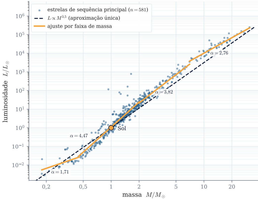
Figura 21: Relação massa-luminosidade da sequência principal. Cada ponto é uma componente de binária eclipsante destacada com massa e raio medidos diretamente; a luminosidade vem de L = 4\pi R^2 \sigma T_{\text{eff}}^4 . Em escala log-log a relação é quase uma reta, o que significa uma lei de potência L \propto M^\alpha : pequenas mudanças de massa produzem grandes mudanças de luminosidade e, portanto, de tempo de vida. O expoente único \alpha = 3,5 (tracejado) é uma boa aproximação de trabalho, mas o ajuste por faixas mostra que \alpha varia de \sim 1,7 nas anãs vermelhas a \sim 4,5 perto da massa solar e volta a cair nas estrelas mais massivas, onde a pressão de radiação domina. Dados: Eker et al. (2018), MNRAS 479, 5491 (via VizieR).
