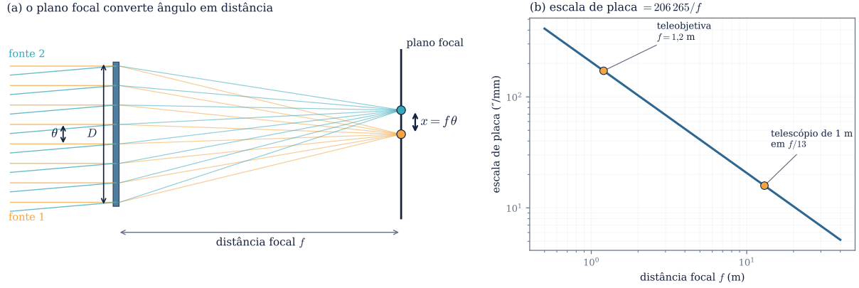
Figura 14: Como um telescópio converte direção em posição. (a) Fontes no infinito chegam como frentes de onda planas; o espelho concentra cada direção em um ponto do plano focal. Duas fontes separadas por um ângulo \theta produzem imagens separadas por x = f\theta — a distância focal f é o fator de conversão, e a abertura D não entra nesta relação. (b) A escala de placa, em segundos de arco por milímetro, é 206\,265/f [mm]: quanto maior a distância focal, menos céu cabe em cada milímetro do detector.
