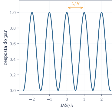
(b) franjas: um período a cada \delta\theta = \lambda/B
