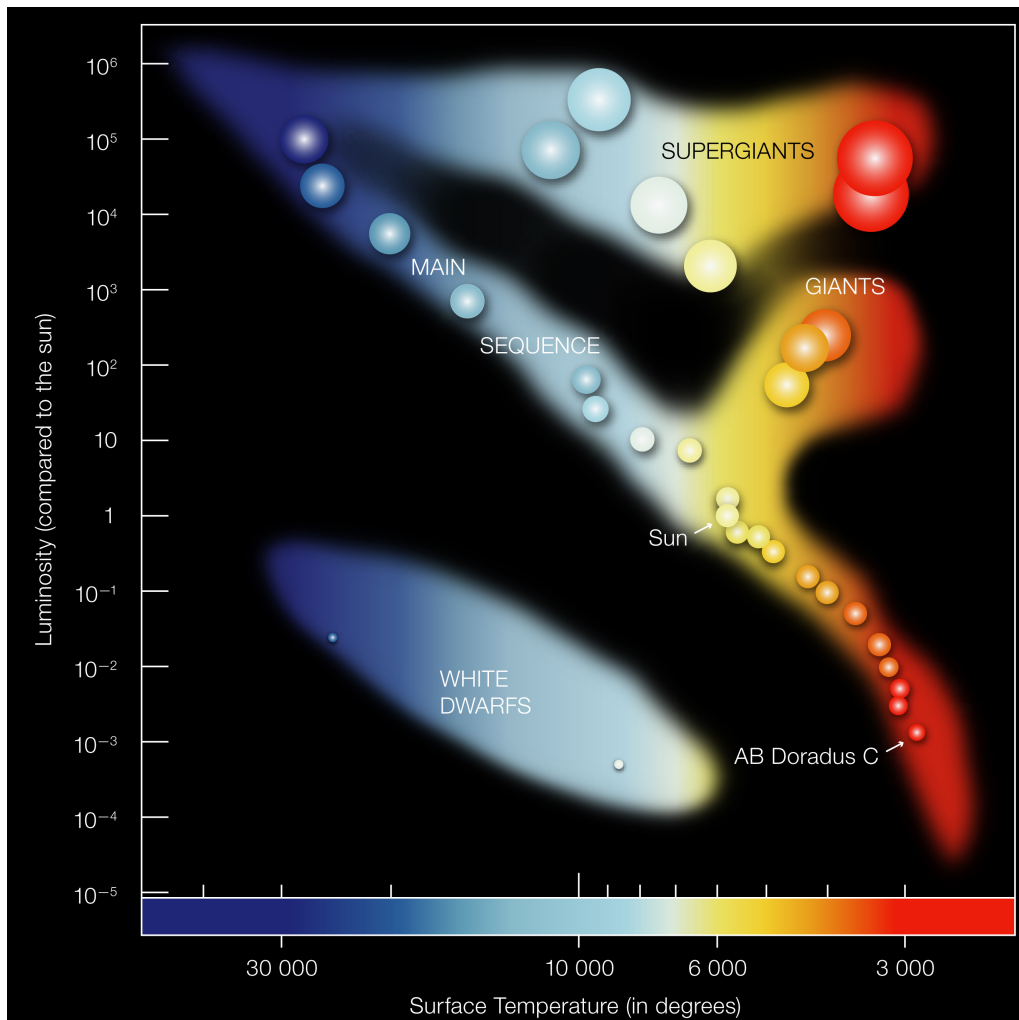
Figura 20: Diagrama Hertzsprung-Russell. Luminosidade (em unidades solares) contra temperatura efetiva, com o eixo de temperatura crescendo para a esquerda. A faixa diagonal é a sequência principal ( main sequence ); acima e à direita estão gigantes ( giants ) e supergigantes ( supergiants ), frias mas luminosas por terem raios enormes; abaixo e à esquerda estão as anãs brancas ( white dwarfs ), quentes mas pouco luminosas por terem raios pequenos. O tamanho dos círculos indica o raio relativo das estrelas. A posição de uma estrela combina temperatura, luminosidade, raio e estágio evolutivo. Crédito: ESO, licença CC BY 4.0 (eso0728c).
