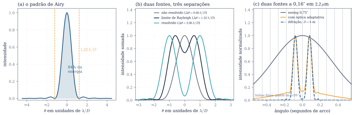
Figura 15: A imagem de uma fonte pontual. (a) O padrão de Airy de uma abertura circular ideal, não obstruída: cerca de 84% da energia cai dentro do primeiro anel escuro, em 1,22 \lambda/D . (b) Duas fontes de igual brilho, somadas em intensidade, para três separações. No critério de Rayleigh o vale entre os picos é raso mas existe; abaixo dele as duas fontes aparecem como uma só. (c) As mesmas duas fontes, separadas por 0,16'' em 2,2 \mu\text{m} , vistas por um telescópio de 8 m: sob seeing de 0,75'' a dupla some; com óptica adaptativa parcial reaparece sobre um halo residual. As linhas verticais são uma grade de pixels de 0,09'' , próxima da amostragem de Nyquist nesse comprimento de onda.
