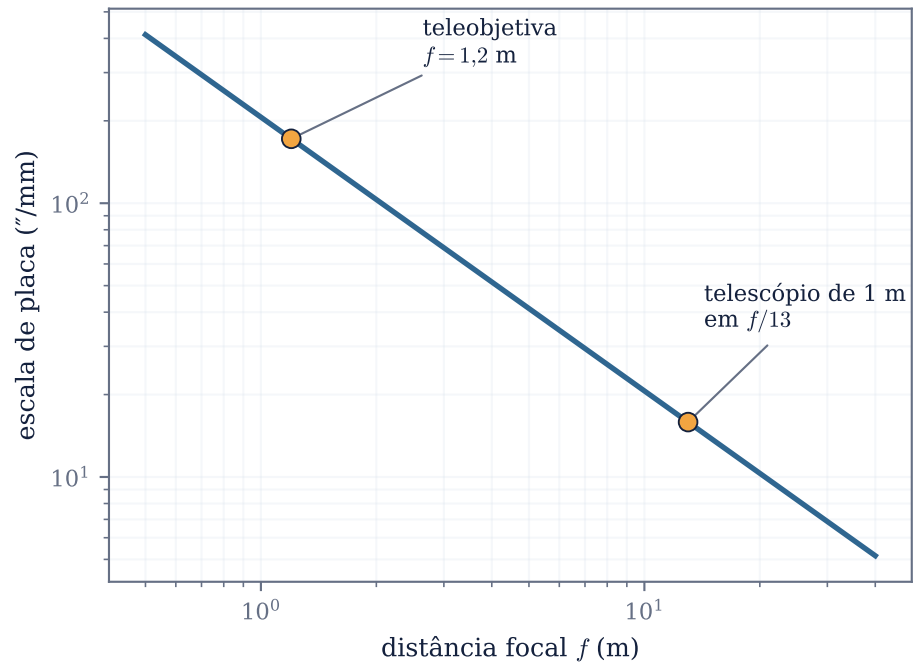
(b) escala de placa = 206\,265/f
