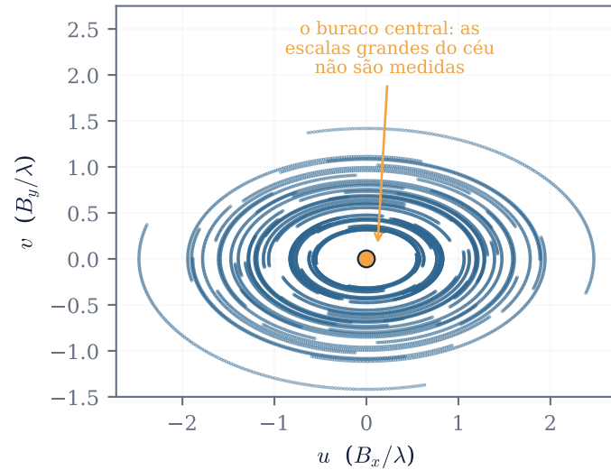
(c) o que a rotação da Terra amostra
