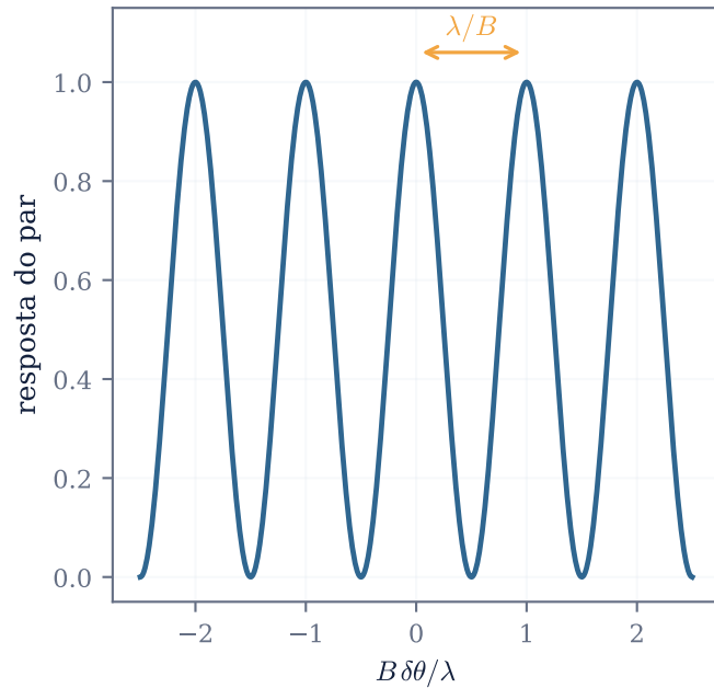
(b) franjas: um período a cada \delta\theta = \lambda/B
