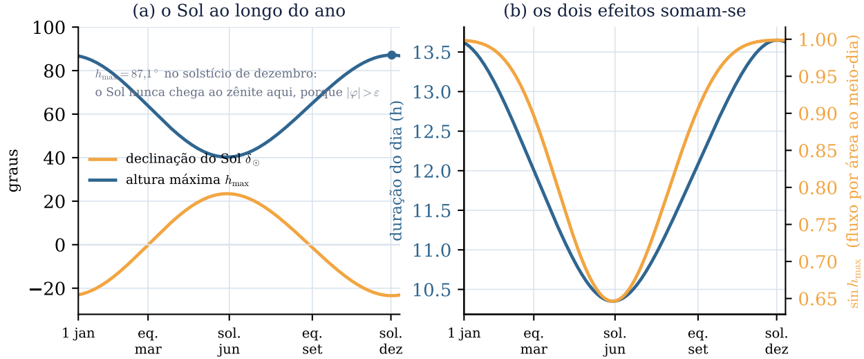
Figura 3: Por que existem estações, em números, para Joinville. (a) A declinação do Sol varia entre \pm\varepsilon ao longo do ano, e com ela a altura máxima h_{\max} = 90^\circ - |\varphi - \delta_\odot| . Como |\varphi| = 26,3^\circ excede a obliquidade, o Sol nunca alcança o zênite aqui: no solstício de dezembro ele para a 87,1^\circ . (b) Os dois efeitos caminham juntos e no mesmo sentido: no verão o dia dura mais (13,6 h contra 10,4 h no inverno) e cada metro quadrado recebe mais fluxo ao meio-dia, porque \sin h_{\max} é maior. É a soma dos dois, e não a distância ao Sol, que produz as estações.
