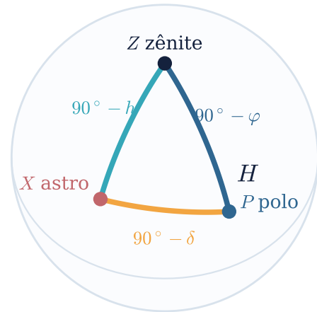
(b) o triângulo esférico PZX
