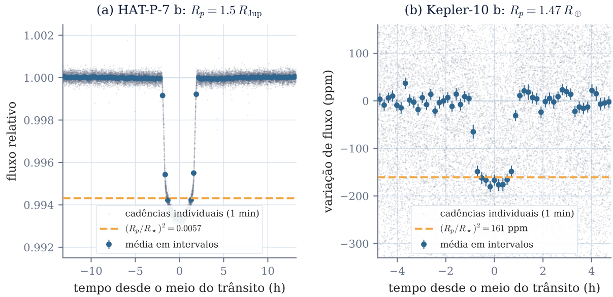
Figura 17: Curvas de luz de trânsito reais, medidas pelo Kepler. Fotometria de cadência curta (um ponto por minuto), dobrada no período orbital; os pontos cinza são cadências individuais e os círculos azuis são médias em intervalos de tempo. A linha tracejada não é ajuste algum: é a profundidade prevista por (R_p/R_\star)^2 com o raio do planeta e o raio da estrela medidos independentemente. (a) HAT-P-7 b, um Júpiter quente diante de uma estrela de 2 R_\odot : a queda é de 0,57% e o fundo achatado mostra o planeta inteiramente projetado sobre o disco estelar. (b) Kepler-10 b, um planeta rochoso de 1,5 R_\oplus : a queda é de apenas 161 partes por milhão, ou seja, 35 vezes menor, exatamente como a razão dos raios ao quadrado prevê. É a mesma física nas duas escalas, e é por isso que a estatística de exoplanetas nasceu dominada por planetas grandes. Dados: arquivo público do Kepler (MAST); efemérides do NASA Exoplanet Archive.
