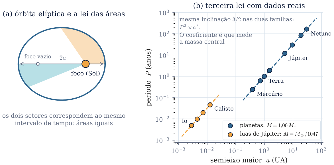
Figura 9: As leis de Kepler. (a) Órbita de excentricidade 0,55 obtida resolvendo a equação de Kepler M = E - e \sin E . O corpo central ocupa um foco, o outro fica vazio, e os dois setores sombreados — percorridos no mesmo intervalo de tempo — têm a mesma área: perto do periélio o planeta corre mais e cobre um ângulo grande com raio curto; perto do afélio faz o oposto. (b) A terceira lei com dados tabelados: os oito planetas em torno do Sol e os quatro satélites galileanos em torno de Júpiter. As duas famílias caem sobre retas de mesma inclinação 3/2 mas coeficientes diferentes, e é o coeficiente que carrega a física: aplicando M = 4\pi^2 a^3 / GP^2 aos planetas obtém-se 1,00 M_{\odot} ; aplicando às luas, 1,90 \times 10^{27} \text{ kg} , a massa de Júpiter, cerca de M_{\odot}/1047 . A mesma lei, medindo dois corpos centrais diferentes.
