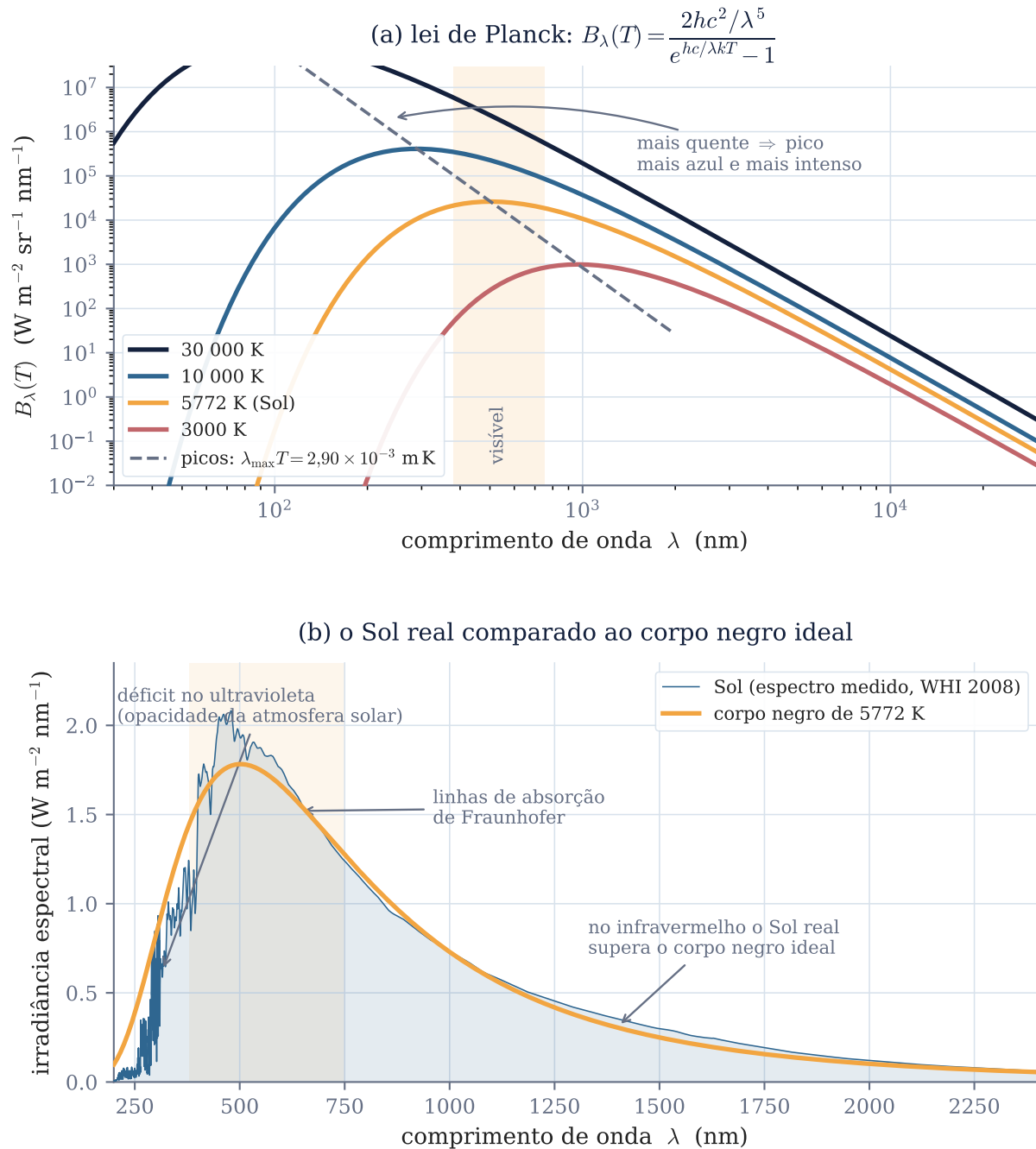
Figura 10: Corpo negro: o ideal e o real. (a) Curvas calculadas diretamente da lei de Planck para quatro temperaturas. Em escala log-log o efeito é duplo: o pico se desloca para comprimentos de onda menores (lei de Wien, tracejado ligando os máximos) e toda a curva sobe, porque o fluxo integrado cresce com T^4 (lei de Stefan-Boltzmann). Note que nenhuma curva cruza outra: uma estrela mais quente emite mais em todo comprimento de onda, e não apenas no azul. (b) O espectro solar realmente medido acima da atmosfera terrestre, comparado ao corpo negro de 5772 K com o mesmo raio e distância. O envelope é bem reproduzido, mas os desvios são grandes e informativos: entre 200 e 400 nm o Sol emite apenas 65% do previsto, porque a opacidade cresce no ultravioleta e a radiação escapa de camadas mais altas e frias; no visível o espectro é recortado pelas linhas de absorção de Fraunhofer; entre 1400 e 2400 nm a emissão real supera a ideal em cerca de 19%. Corpo negro é um ponto de partida, não uma descrição completa. Dados do painel (b): Whole Heliosphere Interval reference spectrum (SORCE/TIMED), LASP/LISIRD, Universidade do Colorado.
