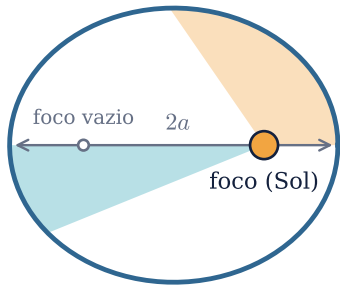
(a) órbita elíptica e a lei das áreas
