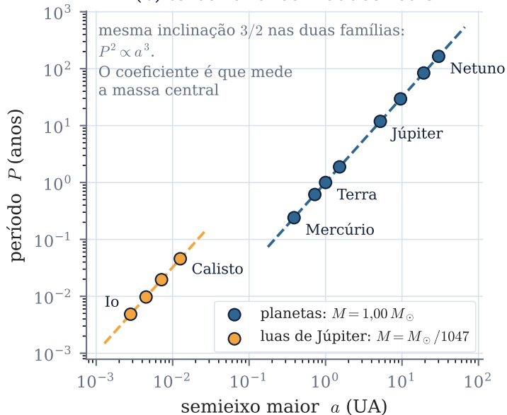
(b) terceira lei com dados reais
