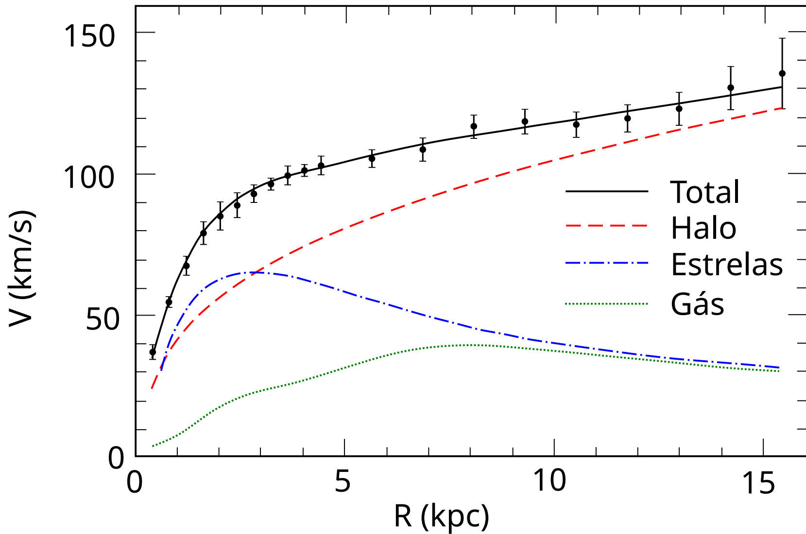
(b) galáxia M 33
