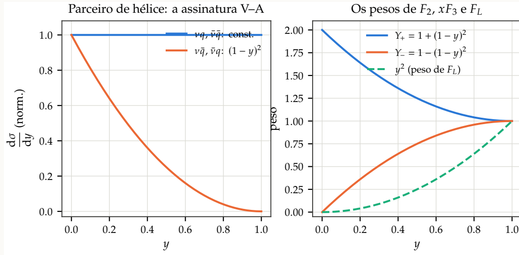
Figura 3.1: Os pesos cinemáticos da eq. (3.17). À direita, Y_+ multiplica F_2 , Y_- multiplica xF_3 e y^2 multiplica F_L : em y pequeno só F_2 sobrevive, e é por isso que a seção de choque reduzida medida a baixo y é essencialmente F_2 . À esquerda, a distribuição em y prevista pelo modelo de pártons (capítulo 4) para quarks e antiquarks.
