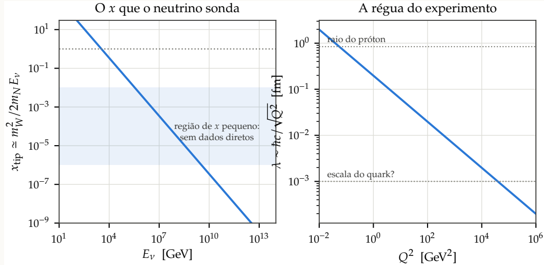
Figura 1.1: À esquerda, a fração de momento x que um neutrino de energia E_\nu tipicamente sonda; à direita, a resolução espacial associada a Q^2 . Um neutrino de 10^9 GeV enxerga pártons com x \sim 10^{-6} — três ordens de grandeza abaixo do menor x jamais medido.
