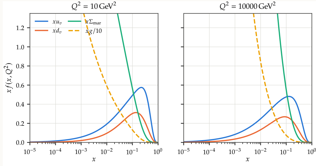
Figura 4.1: Distribuições de pártons do próton, HERAPDF2.0 LO [1], em duas escalas. Note o que a evolução faz: em Q^2 maior, a valência encolhe e migra para x pequeno, enquanto o mar e o glúon explodem. O glúon está dividido por 10 para caber no gráfico.
