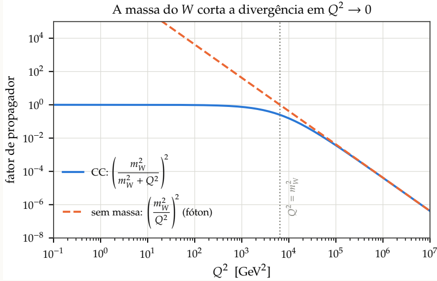
Figura 6.1: O fator de propagador. Para Q^2 \ll m_W^2 ele é constante — a interação é efetivamente pontual, e recupera-se a teoria de Fermi. Para Q^2 \gg m_W^2 ele cai como 1/(Q^2)^2 e sufoca a seção de choque. A transição em Q^2 = m_W^2 é o que impede \sigma_{\nu N} de crescer linearmente para sempre.
