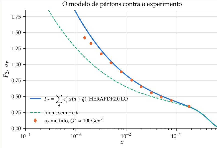
Figura 5.2: A eq. (4.8) avaliada com as PDFs HERAPDF2.0 LO, contra a seção de choque reduzida medida em Q^2 \approx 100 \text{ GeV}^2 [1]. A curva tracejada mostra o mesmo cálculo omitindo charm e bottom: em x pequeno, os quarks pesados respondem por quase 30% de F_2 . Não é um ajuste — os pontos e a curva vêm da mesma publicação, mas a curva é a fórmula do modelo de pártons com as PDFs postas dentro.
