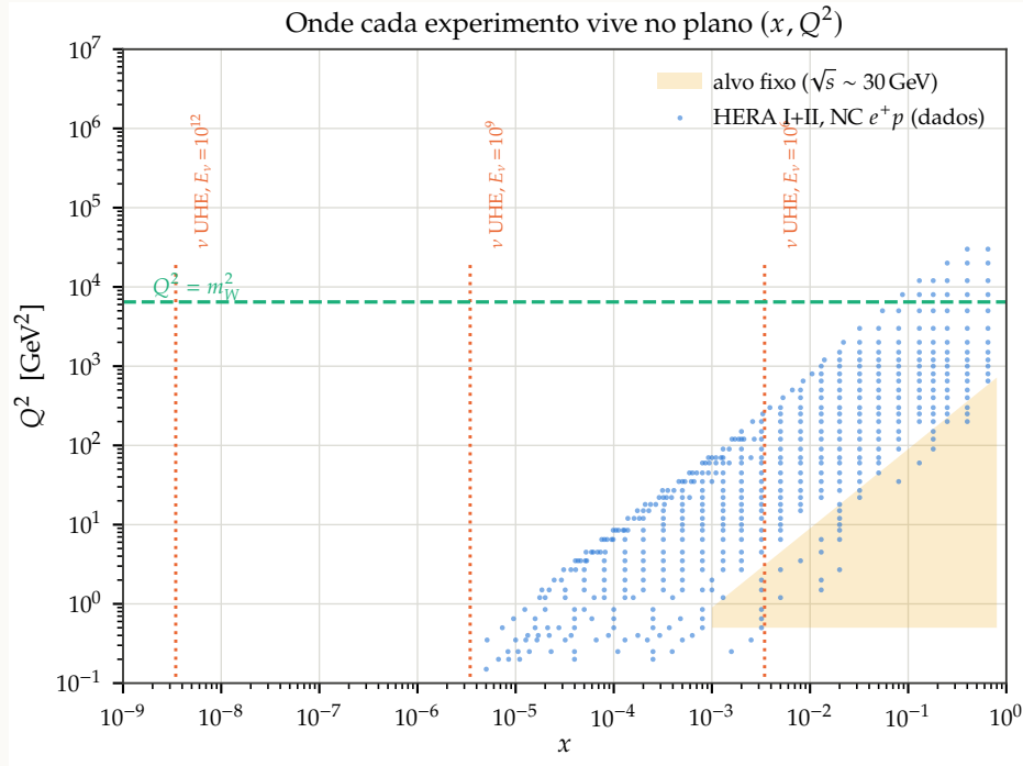
Figura 2.2: O plano (x, Q^2) . Os pontos são as 485 medidas combinadas de H1 e ZEUS para corrente neutra e^+p [1]; a faixa clara é a região típica de experimentos de alvo fixo. As linhas pontilhadas marcam o x que um neutrino de energia E_\nu sonda quando o propagador do W fixa Q^2 \sim m_W^2 . A distância entre os dados e essas linhas é o problema central da física de neutrinos UHE.
