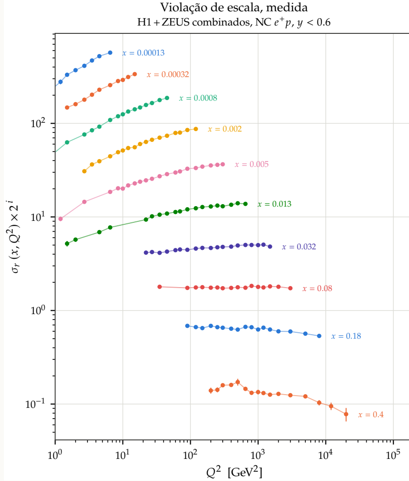
Figura 5.1: A previsão de DGLAP contra a natureza. Cada série é um x fixo, deslocada verticalmente por 2^i para não se sobrepor. Dados combinados de H1 e ZEUS, corrente neutra e^+p , \sqrt{s} = 318 GeV, restritos a y < 0,6 para que \sigma_r \approx F_2 [1]. Em x pequeno a seção de choque cresce com Q^2 ; em torno de x \approx 0,13 ela é plana (escalonamento exato!); em x grande ela decrece . É exatamente o padrão que a eq. (5.2) prevê: aumentar Q^2 resolve emissões, o que desloca pártons de x grande para x pequeno.
