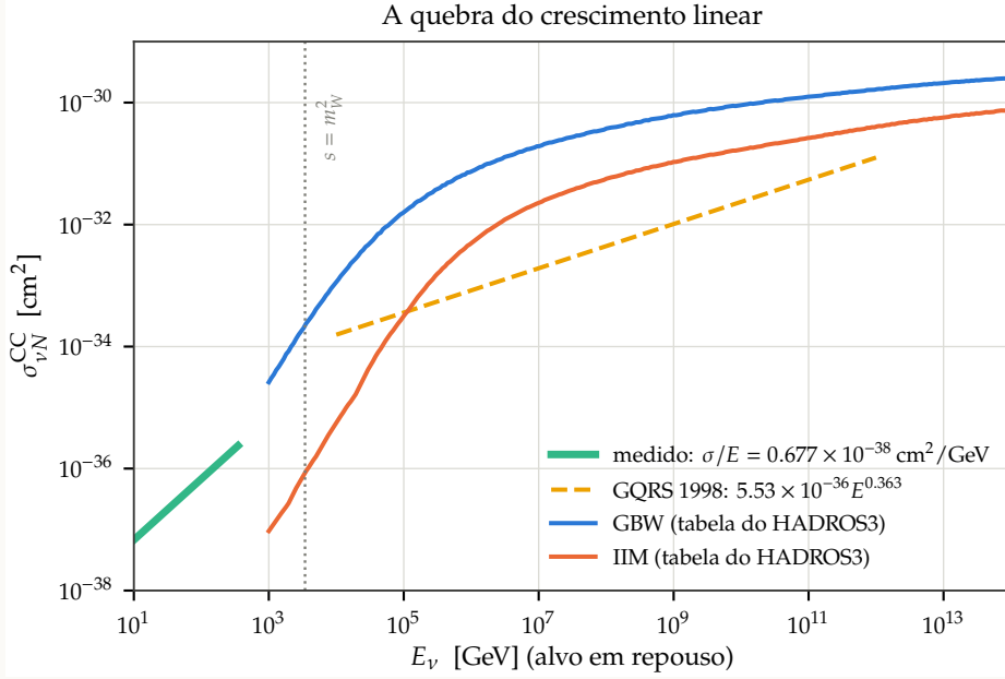
Figura 6.2: A seção de choque \nu N de corrente carregada em treze ordens de grandeza de energia. O segmento grosso é o regime linear medido em aceleradores [24]; a linha tracejada é a parametrização de Gandhi et al. [25], na faixa em que os autores a declararam válida; as duas curvas cheias são as tabelas GBW e IIM embarcadas no HADROS3.
