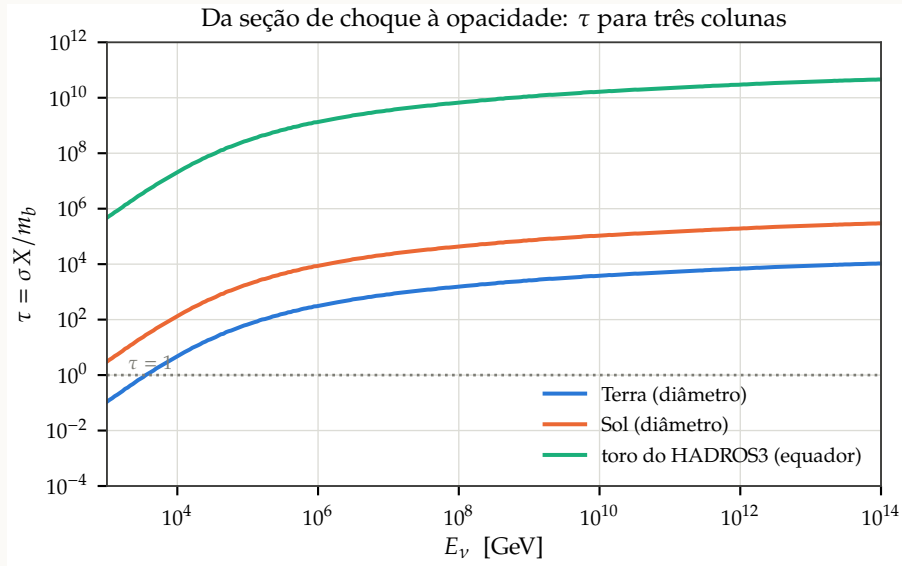
Figura 6.3: A eq. (6.4) para três colunas de matéria, usando a tabela GBW. A Terra fica opaca em torno de algumas dezenas de TeV — e é exatamente essa opacidade que o IceCube usou para medir \sigma_{\nu N} [29]. O toro do HADROS3, com a configuração padrão, é opaco por nove ordens de grandeza no plano equatorial.
