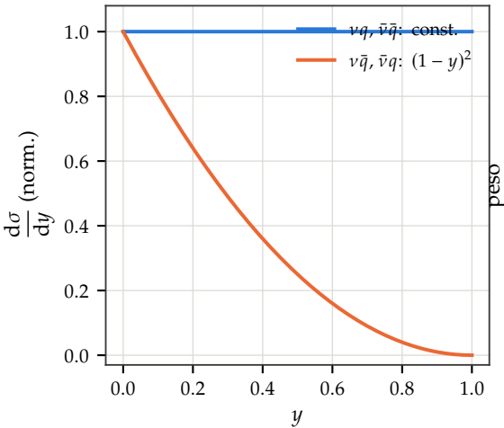
Parceiro de hélice: a assinatura V-A
