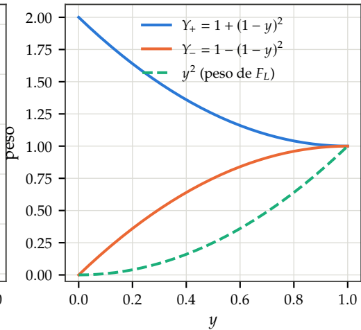
Os pesos de F_2 , x F_3 e F_L
