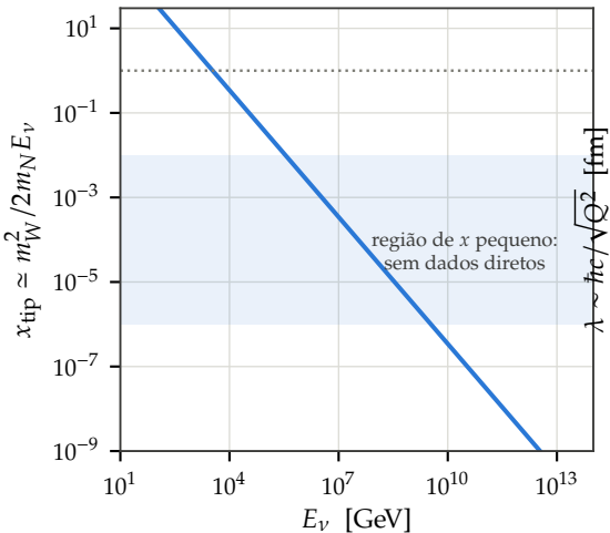
O x que o neutrino sonda
