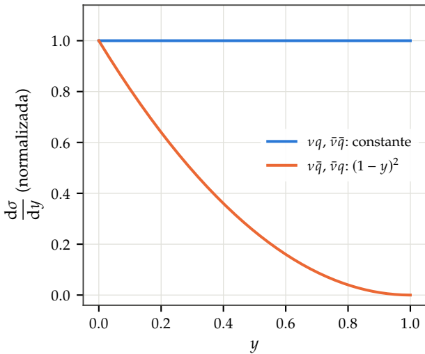
Parceiro de hélice: a assinatura V-A
