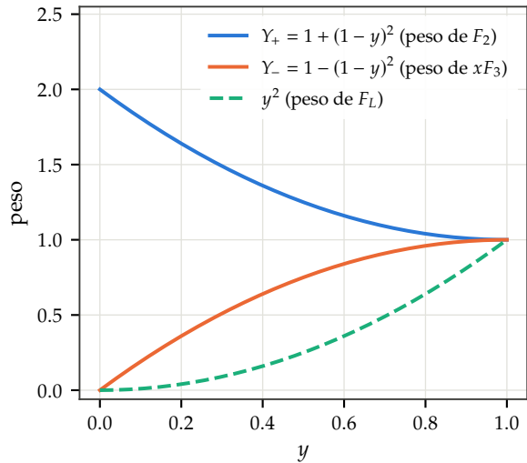
Os pesos de F_2 , xF_3 e F_L
