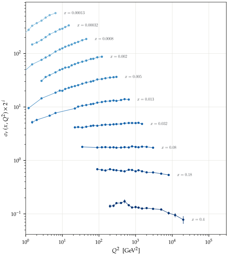
Violação de escala, medida H1 + ZEUS combinados, NC e^+p , y < 0.6
