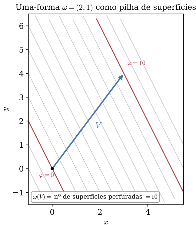
Figura 3.1. A 1-forma \omega = (2, 1) representada como uma pilha de retas (superfícies de nível de \varphi = 2x + y , espaçadas de \Delta\varphi = 1 ). O vetor V = (3, 4) vai de \varphi = 0 a \varphi = 10 , perfurando exatamente 10 retas – por isso \omega(V) = 10 . Esses são os mesmos \omega e V do Exemplo 3.1.
