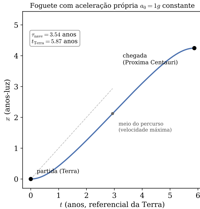
Figura 2.5. Trajetória no plano (t, x) do referencial da Terra para uma nave com aceleração própria constante a_0 = 1g , acelerando até o meio do percurso e desacelerando depois, para alcançar Proxima Centauri ( D = 4,25 anos-luz) em repouso. A reta tracejada é o cone de luz ( x = t ): a trajetória nunca a alcança.
