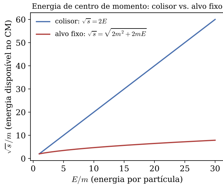
Figura 2.2. Energia disponível no referencial de centro de momento, \sqrt{s} , em função da energia E de cada partícula (mesma massa m nos dois casos). No colisor, \sqrt{s} = 2E cresce linearmente com E . No alvo fixo, \sqrt{s} = \sqrt{2m^2 + 2mE} cresce apenas com \sqrt{E} para E \gg m . A defasagem entre as duas curvas é exatamente a energia “desperdiçada” em manter o centro de momento em movimento no laboratório.
