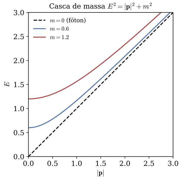
Figura 2.3. Casca de massa E^2 = |\mathbf{p}|^2 + m^2 no plano (|\mathbf{p}|, E) . Para m > 0 a curva é um ramo de hipérbole que nunca toca a reta E = |\mathbf{p}| : por maior que seja o momento, E > |\mathbf{p}| sempre. Para m = 0 a casca degenera na própria reta E = |\mathbf{p}| – não há “folga” entre energia e momento para o fóton.
