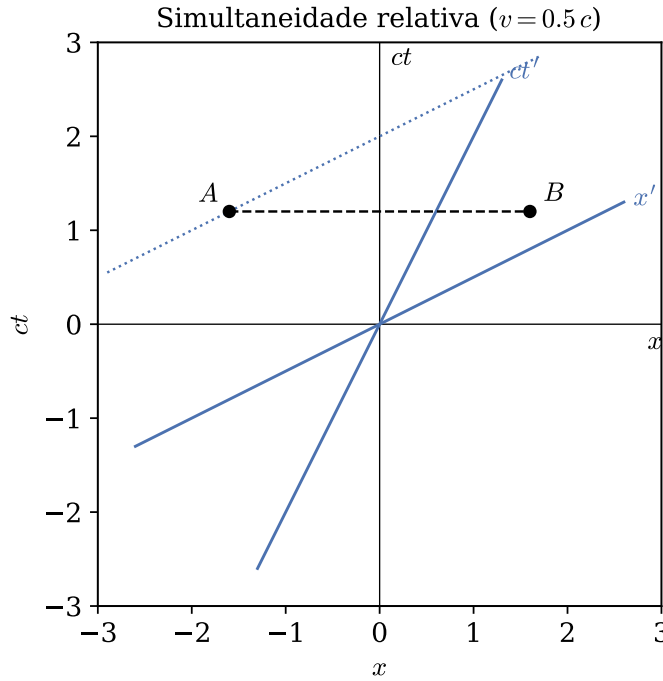
Figura 1.3. Diagrama de Minkowski: os eixos ct' e x' de S' aparecem inclinados em relação aos eixos de S pelo mesmo ângulo \arctan v . A reta tracejada liga dois eventos A e B simultâneos em S (mesma ct ); a reta pontilhada é a reta de simultaneidade de S' passando por A – ela não contém B .
