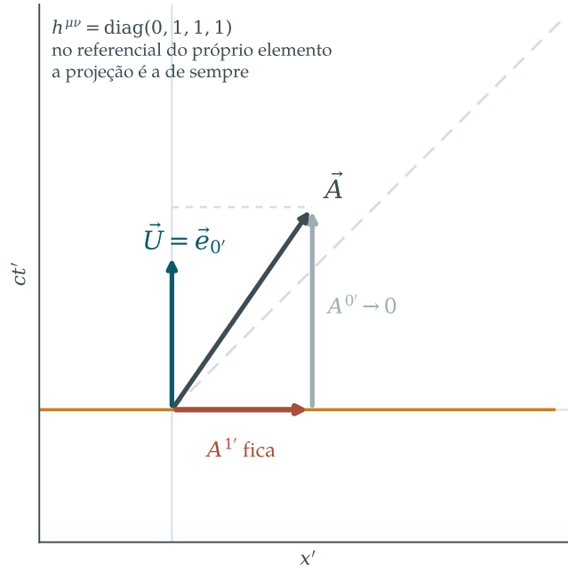
Figura 4.6. O mesmo \vec{A} visto do MCRF, onde \vec{U} aponta para cima e a reta ortogonal é o eixo x' . Ali a projeção oblíqua das duas figuras anteriores vira a projeção perpendicular de sempre: a perna temporal A^{0'} é descartada e a espacial A^{1'} sobrevive inteira.
