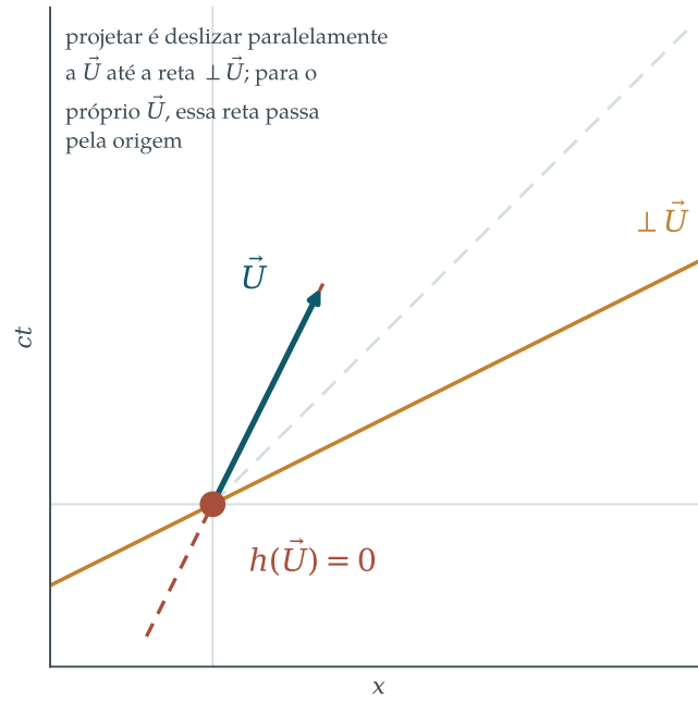
Figura 4.4. Projetar é deslizar paralelamente a \vec{U} até a reta ortogonal a ele — que é a reta de simultaneidade do elemento, e o reflexo de \vec{U} na linha de luz, como no Capítulo 2. Aplicada ao próprio \vec{U} , a reta de deslizamento passa pela origem, e a sombra é o ponto zero: h(\vec{U}) = 0 .
