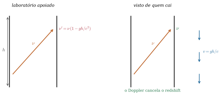
Figura 5.2. A mesma torre, vista do referencial que cai livremente. À esquerda, o laboratório apoiado: o fóton sobe e chega com frequência menor. À direita, visto de quem cai: no tempo de voo h/c o referencial adquiriu velocidade gh/c para baixo, e o Doppler correspondente cancela o redshift.
