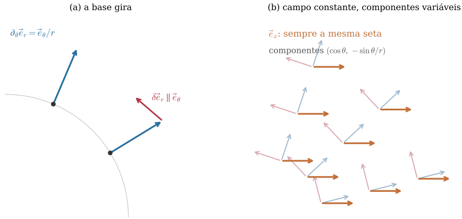
Figura 5.5. À esquerda, a origem geométrica de (5.10): ao avançar \delta\theta , a base inteira gira, e a diferença \vec{e}_r(\theta + \delta\theta) - \vec{e}_r(\theta) aponta na direção de \vec{e}_\theta . À direita, o campo constante \vec{e}_x desenhado sobre bases que giram: a seta é sempre a mesma, as componentes não.
