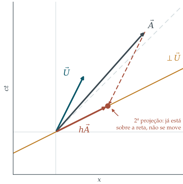
Figura 4.5. O mesmo deslizamento, agora sobre um vetor qualquer: \vec{A} desce paralelamente a \vec{U} e pousa em h\vec{A} , sobre a reta. Repetir a operação não move nada, porque h\vec{A} já está lá — que é o conteúdo geométrico de h^\mu{}_\beta h^\beta{}_\nu = h^\mu{}_\nu .
