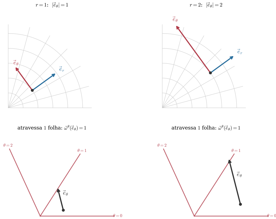
Figura 5.4. A base polar e a base dual em dois pontos de raios diferentes. Em cima, os vetores: \vec{e}_\theta cresce com r . Embaixo, as pilhas das 1-formas: a de \tilde{\omega}^\theta rareia com r , exatamente na proporção inversa. O pareamento \tilde{\omega}^\theta(\vec{e}_\theta) = 1 vale nos dois pontos — a seta mais longa atravessa folhas mais espaçadas, e o produto não muda.
