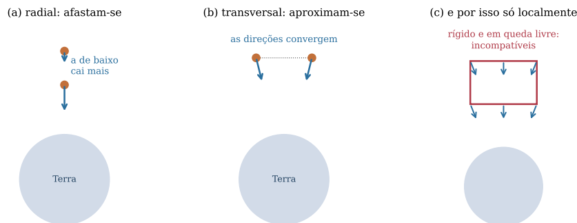
Figura 5.3. Por que um laboratório extenso não permanece inercial. À esquerda, duas partículas separadas radialmente caem para o mesmo centro e se afastam , porque a de baixo é mais acelerada. No meio, separadas transversalmente, elas se aproximam , porque as duas direções de queda convergem. À direita, a consequência: um referencial rígido não pode cair livremente em toda a sua extensão.
