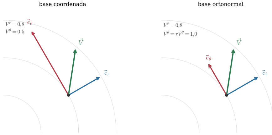
Figura 5.6. O mesmo vetor, no mesmo ponto, decomposto nas duas bases. À esquerda, a base coordenada, com \vec{e}_\theta de comprimento r ; à direita, a base ortonormal, com \vec{e}_\theta de comprimento 1. As componentes diferem pelo fator r de (5.23) — e as unidades também, o que é o ponto.
