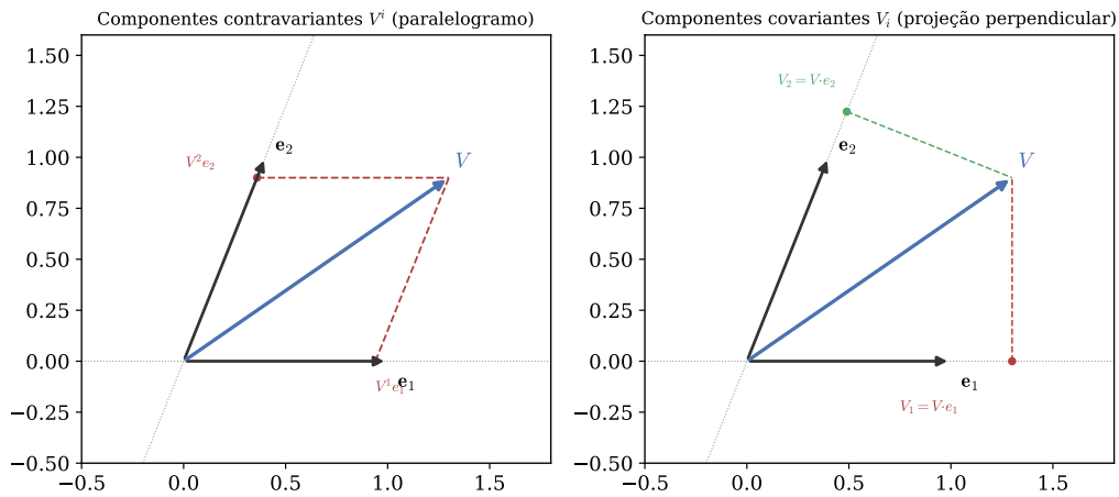
Figura 3.5. O mesmo vetor V , na mesma base oblíqua \{e_1, e_2\} , decomposto de duas maneiras. À esquerda, a regra do paralelogramo dá as componentes contravariantes V^i . À direita, a projeção perpendicular sobre cada eixo, medida em unidades de |\vec{e}_i| , dá as componentes covariantes V_i = V \cdot \vec{e}_i . Numericamente, com e_1 = (1, 0) , e_2 = (0, 4, 1) e V = (1, 3, 0, 9) : V^1 = 0,94 , V^2 = 0,9 , mas V_1 = 1,3 , V_2 = 1,42 .
