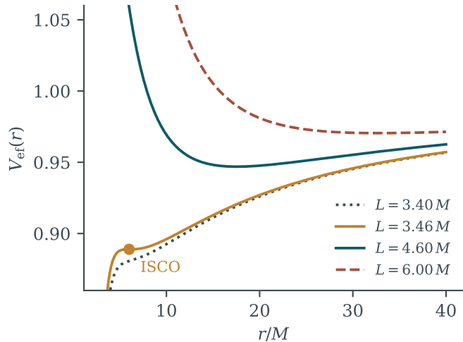
Potencial efetivo
