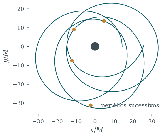
Órbita com p = 20M , e = 0.4
